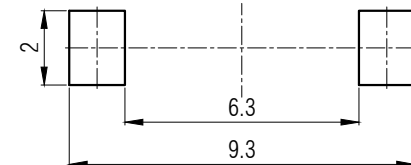
P.C.B. LAYOUT
