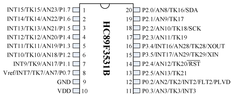
Figure 1-4 SOP20/TSSOP20 引脚配置图
