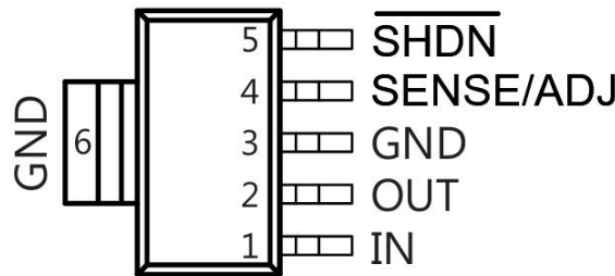
5 引脚 SOT-223 裸露焊盘必须焊接到 PCB 上 图 3 引脚配置(GM12043AKCZ-R7)
