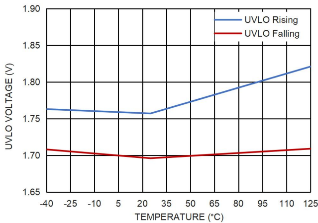
图 14. UVLO 阈值
