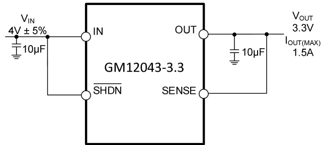
典型应用
