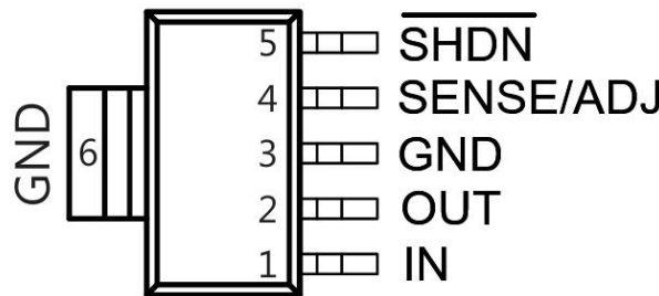
5 引脚 SOT-223 裸露焊盘必须焊接到 PCB 上 图 3 引脚配置(GM12043AKCZ-1-R7)
