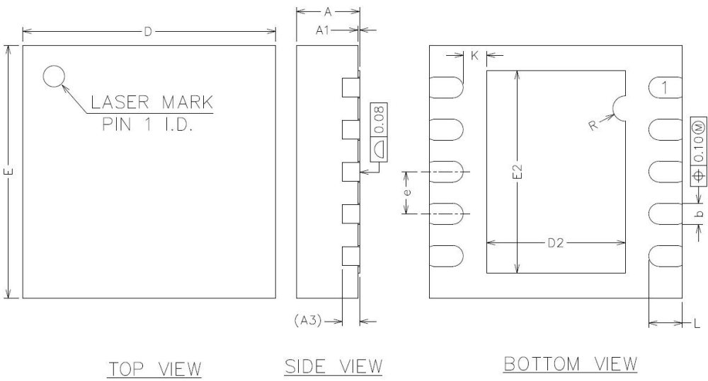
图 26. DFN10 封装 (3mmx3mm)
