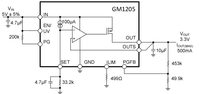
图 23 典型应用
