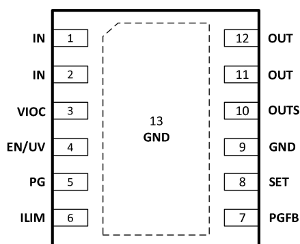
图 3. DFN12 (3mmx3mm GM1205ACPZ-2) 和 PMSOP12 (4mmx4.9mm, GM1205ACPZ-1, 兼容 MSOP-12) 引脚配置(顶视图)
