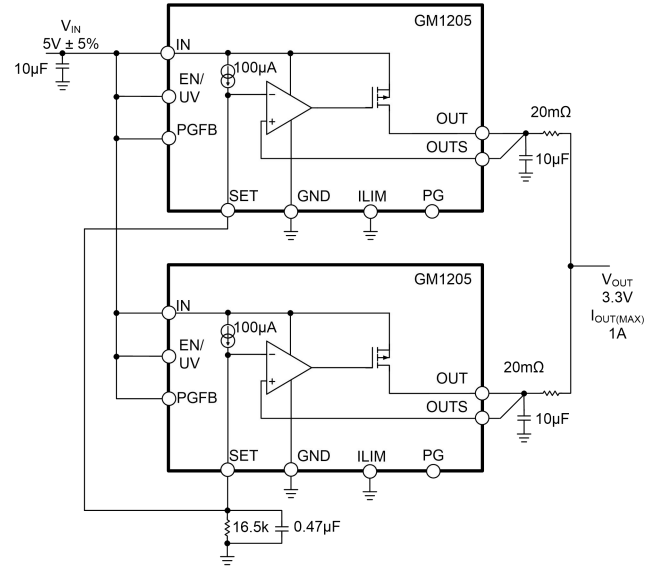
图 24. 并联设备
