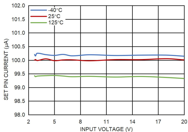
图 5. SET pin 电流和输入电压的关系
