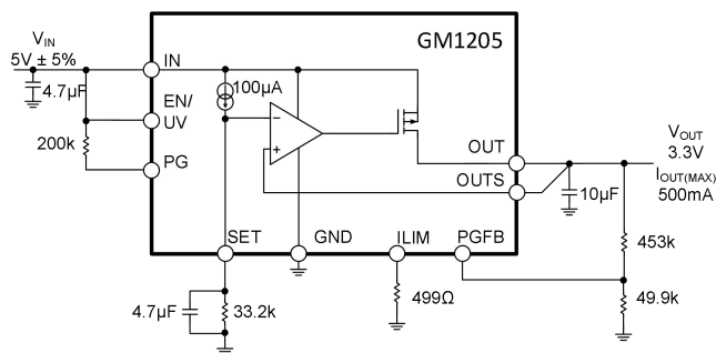
图 1. 典型应用
