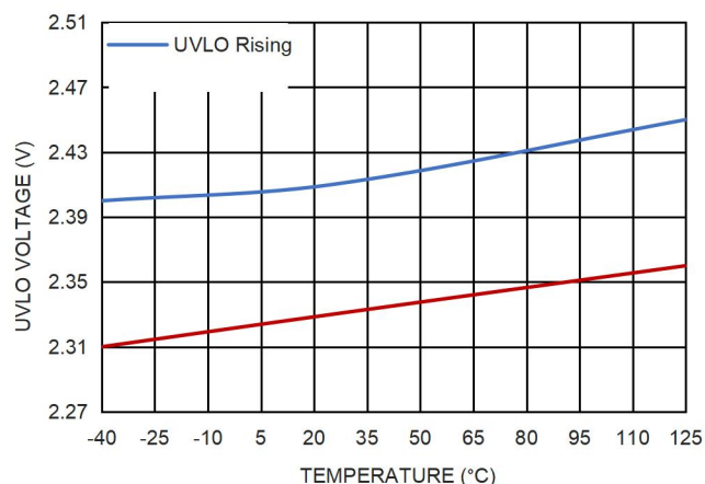
图 14. UVLO 阈值
