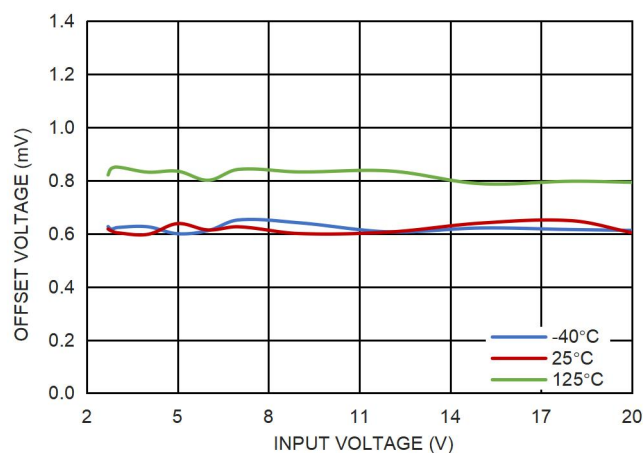
图 7. |V_{OUT}-V_{SET}| 和输入电压的关系, V_{OUT}=1.8V
