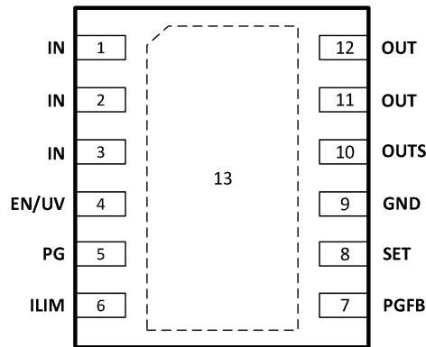
图 4. PMSOP12 (4mmx4.9mm, GM1205ACPZ-3 兼容 MSOP-12) 引脚配置(顶视图)
