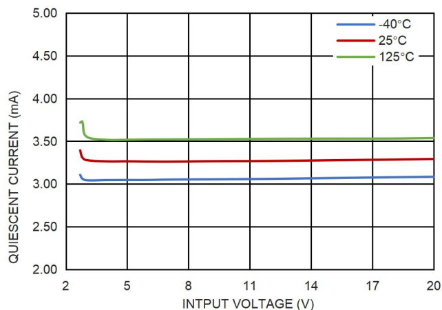
图 11. 静态电流和输入电压的关系, I_{OUT}=10mA
