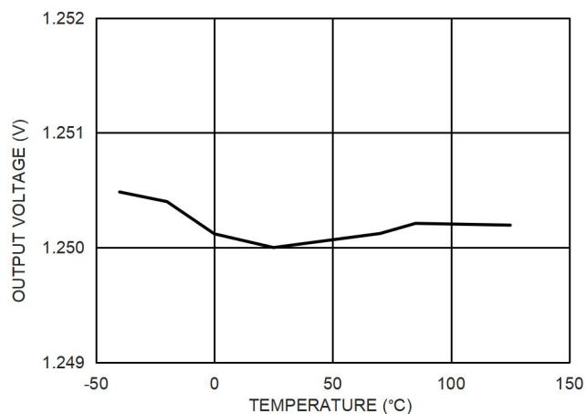
图 5. 1.25V 输出电压和温度的关系
