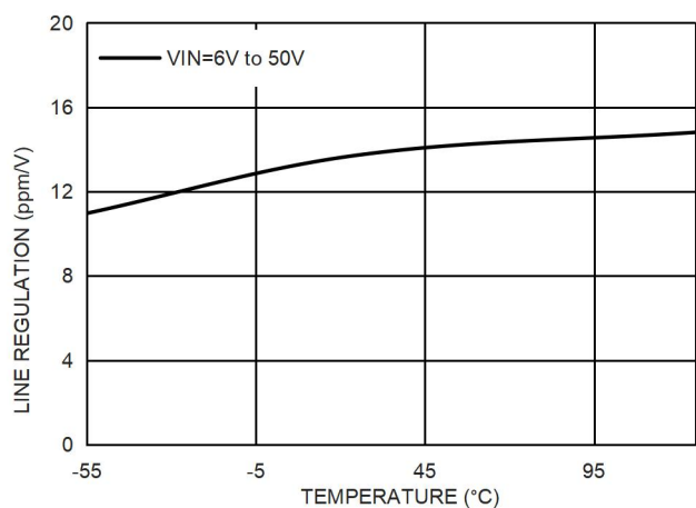
图 15. 输入调整率和温度的关系, V_{OUT}=3.3V
