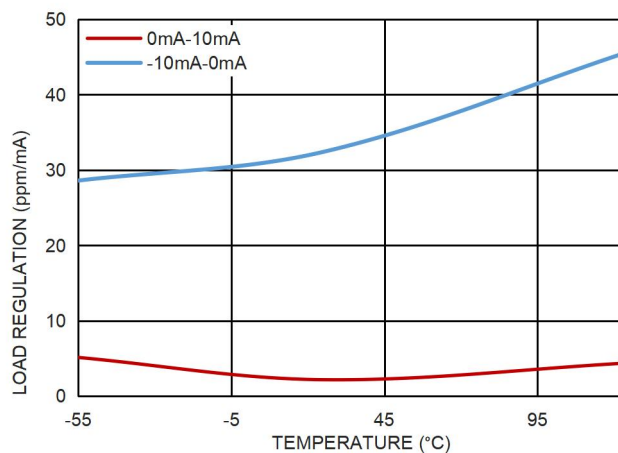
图 10. 负载调整率和温度的关系, V_{OUT}=2.048V
