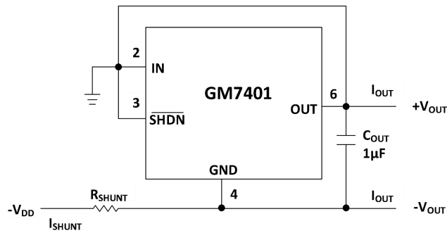
图 26. 负压并联方式
