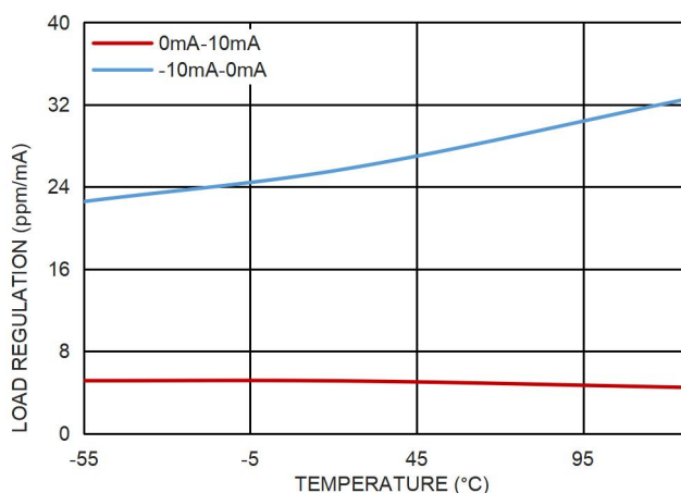
图 11. 负载调整率和温度的关系, V_{OUT}=3.3V
