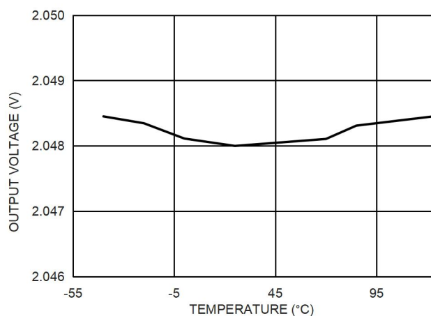
图 6. 2.048V 输出电压和温度的关系
