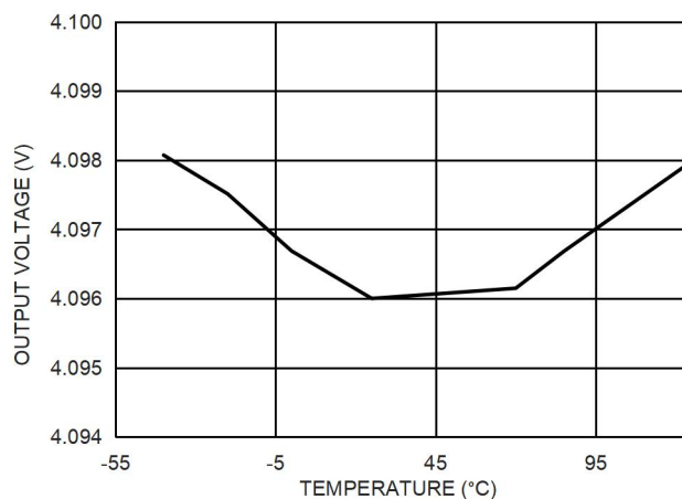
图 8. 4.096V 输出电压和温度的关系
