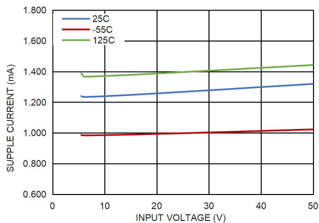
图 19. 输入电流和输入电压的关系, V_{OUT}=3.3V
