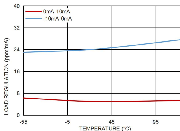
图 12. 负载调整率和温度的关系, V_{OUT}=4.096V
