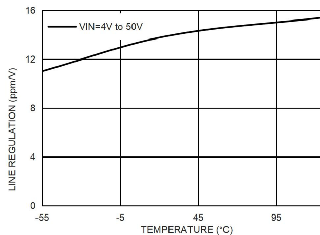
图 14. 输入调整率和温度的关系, V_{OUT}=2.048V
