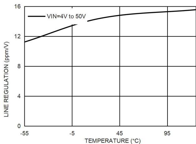
图 13. 输入调整率和温度的关系, V_{OUT}=1.25V
