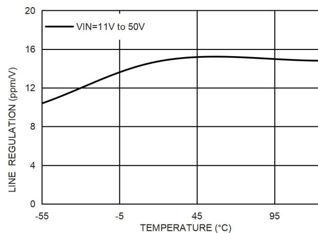
图 16. 输入调整率和温度的关系, V_{OUT}=4.096V
