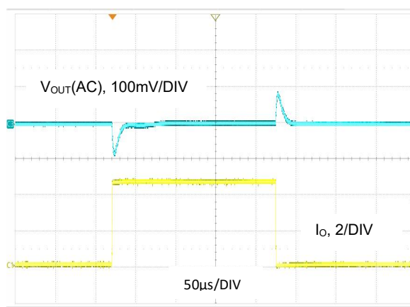
图 30. V_{OUT} = 1.2V , I_O = 0.1A 至 4.5A , FPWM 模式
