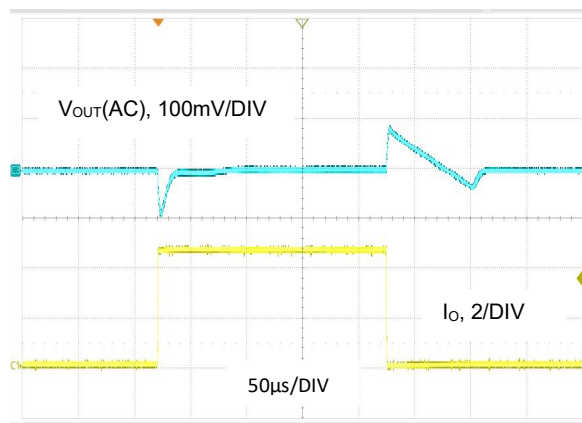
图 31. V_{out} = 1.2V , I_o = 0.1A 至 4.5A , PSM 模式
