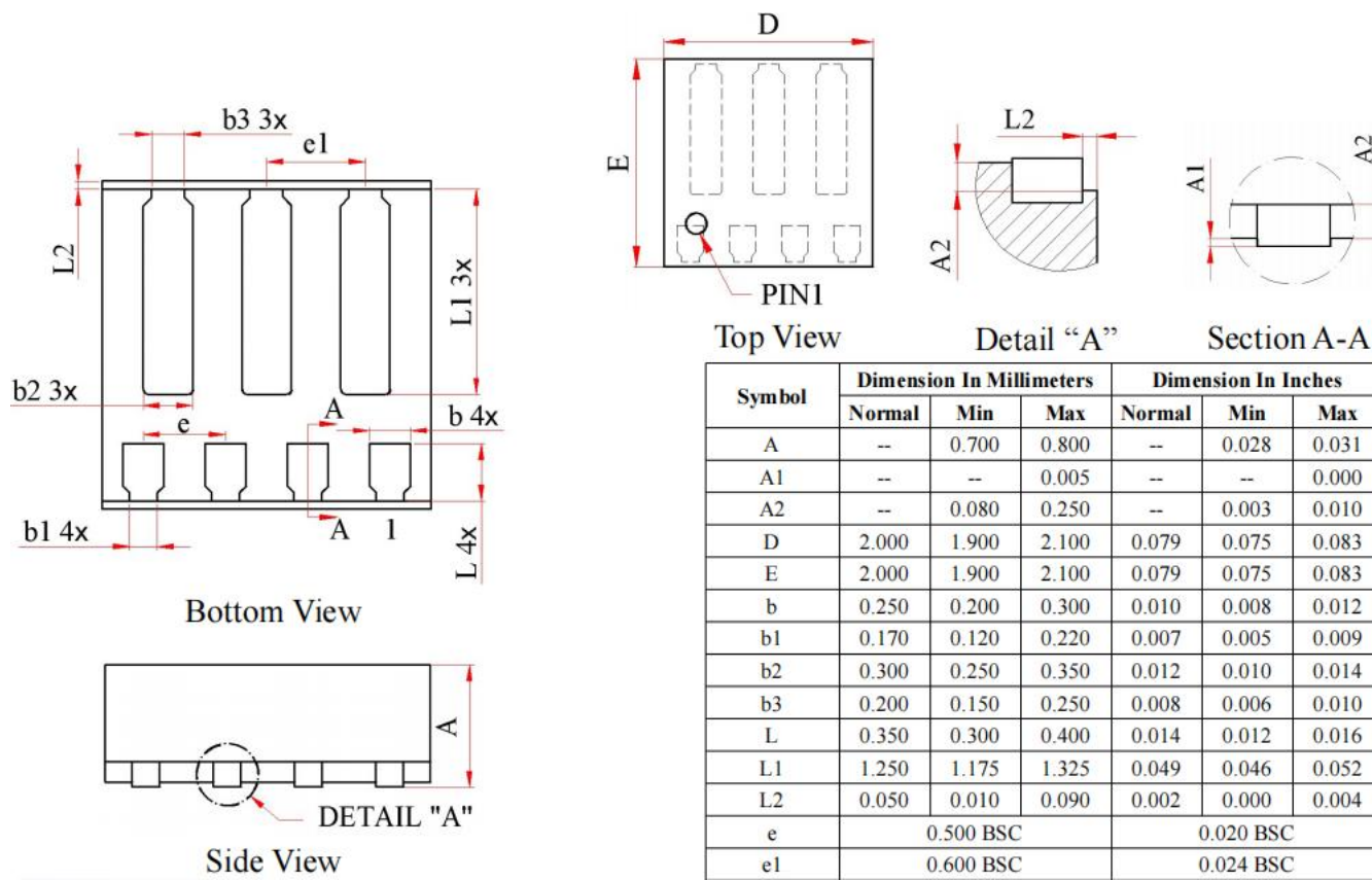
图 44. 7 引脚 LQFN(2mm x 2mm)
