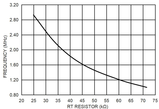
图 19. 频率和 RT 电阻的关系
