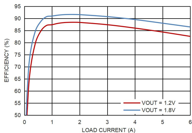
图 13. 效率曲线, V_{IN} = 3.3V , F_{SW} = 4MHz , FPWM
