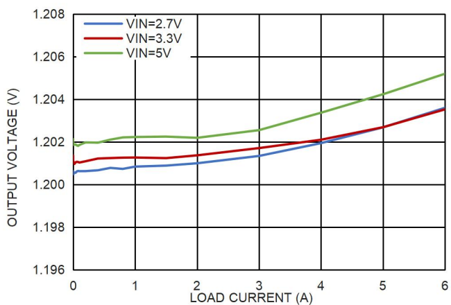
图 21. 输出电压负载调整率, V_{OUT} = 1.2V
