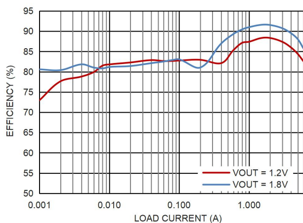
图 9. 效率曲线, V_{IN} = 3.3V , F_{SW} = 4MHz , 低功耗模式
