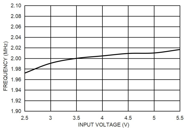
图 18. 频率和输入电压的关系, RT 接高
