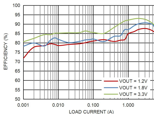
图 10. 效率曲线, V_{IN} = 5V , F_{SW} = 4MHz , 低功耗模式
