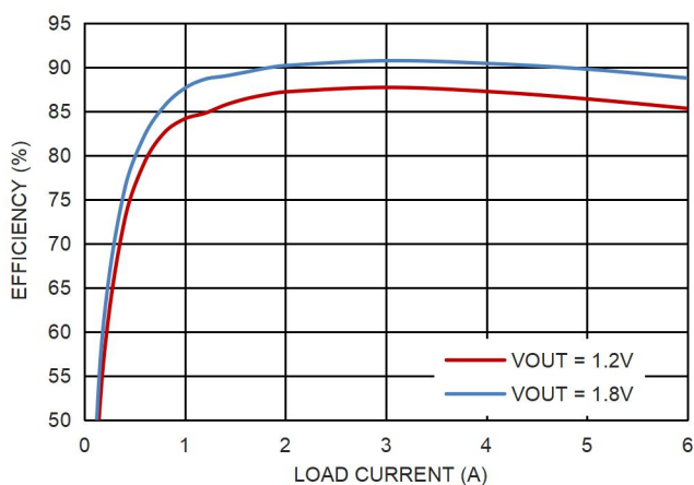
图 14. 效率曲线, V_{IN} = 5V , F_{SW} = 4MHz , FPWM
