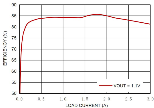
图 15. GM25003 效率曲线, V_{IN} = 3.3V , 低功耗模式
