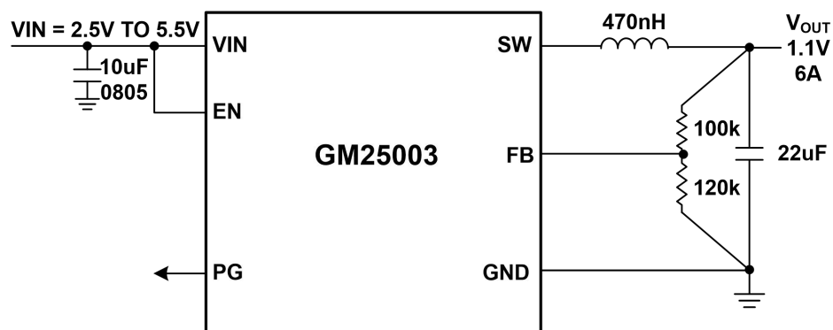
图 41. GM25003, 2.4MHz, V_{IN}=5V , V_{OUT}=1.1V , I_{LOAD}=3A
