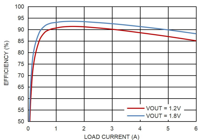
图 11. 效率曲线, V_{IN} = 3.3V , F_{SW} = 2MHz , FPWM
