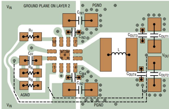
图 34. GM2500 和 GM25001 PCB 推荐布局
