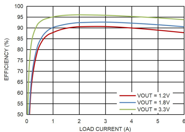
图 12. 效率曲线, V_{IN} = 5V , F_{SW} = 2MHz , FPWM
