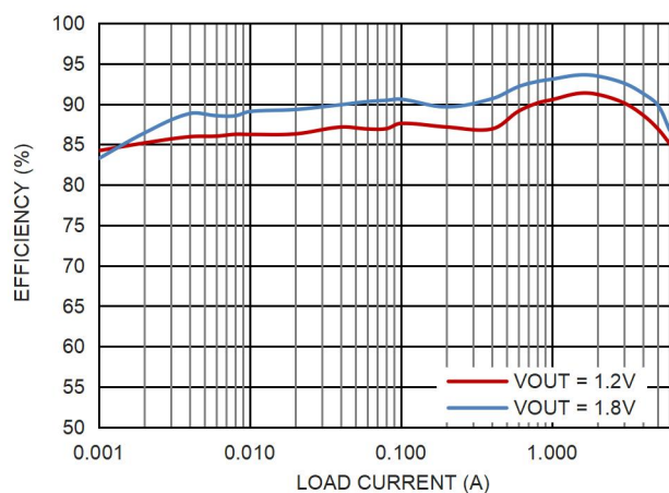
图 7. 效率曲线, V_{IN} = 3.3V , F_{SW} = 2MHz , 低功耗模式
