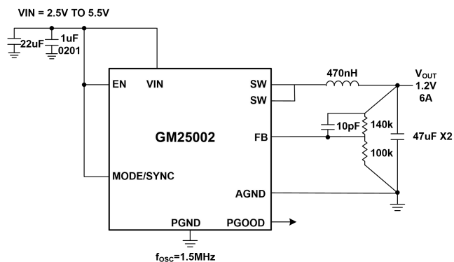
图 2. GM25002 1.5MHz 典型应用
