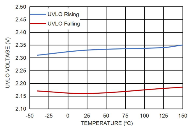
图 24. UVLO 阈值和温度的关系
