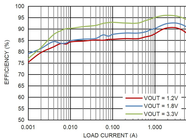
图 8. 效率曲线, V_{IN} = 5V , F_{SW} = 2MHz , 低功耗模式
