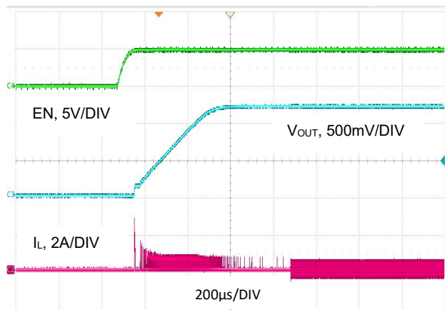
图 25. 启动波形, V_{OUT} = 1.2V , I_O = 10mA
