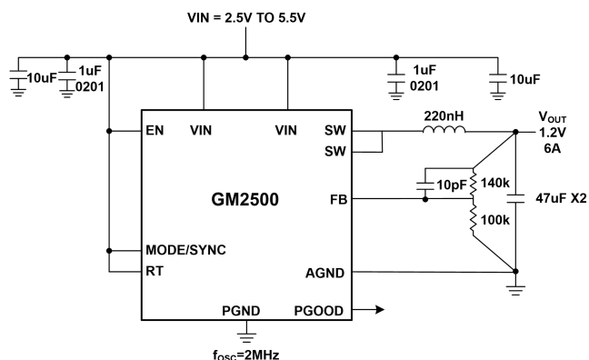
图 1. GM2500 2MHz 典型应用
