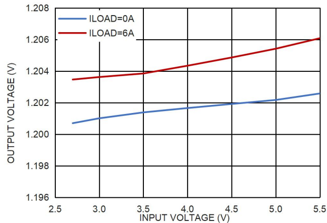
图 22. 输出电压线调整率, V_{OUT} = 1.2V
