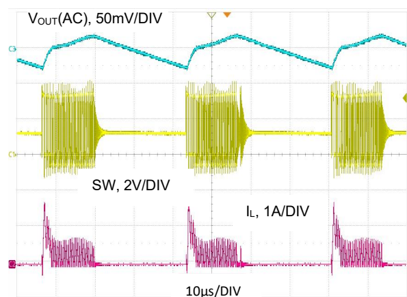
图 29. V_{OUT} = 1.2V , I_O = 10mA , 低功耗模式
