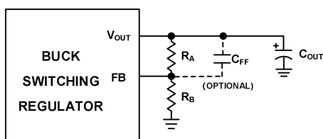
图 33. 反馈电阻网络
