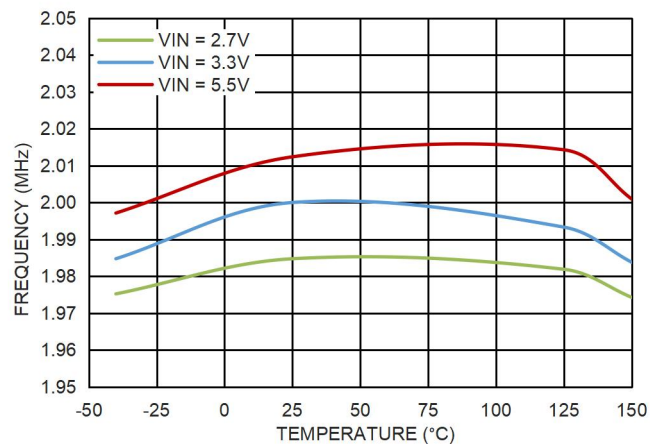
图 20. 频率和温度的关系, RT 接高
