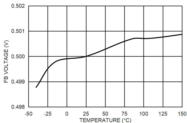
图 17. FB 引脚电压和温度的关系
