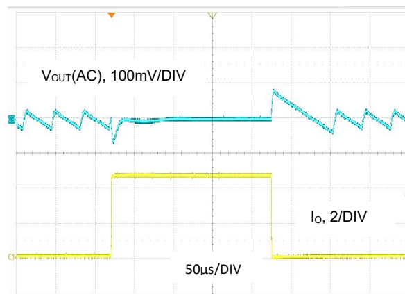
图 32. V_{out} = 1.2V , I_o = 0.1A 至 4.5A , 低功耗模式
