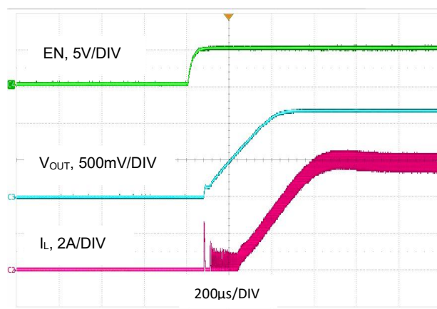
图 26. 启动波形, V_{OUT} = 1.2V , I_O = 6A
