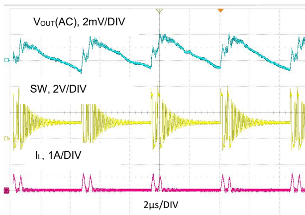
图 28. V_{OUT} = 1.2V , I_O = 100mA , PSM 模式
