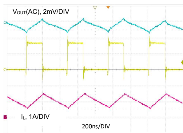
图 27. V_{OUT} = 1.2V , I_O = 1A , FPWM
