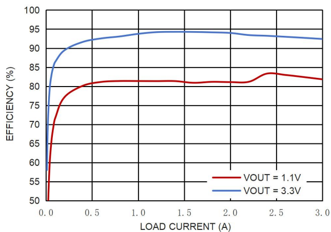
图 16. GM25003 效率曲线, V_{IN} = 5V , 低功耗模式
