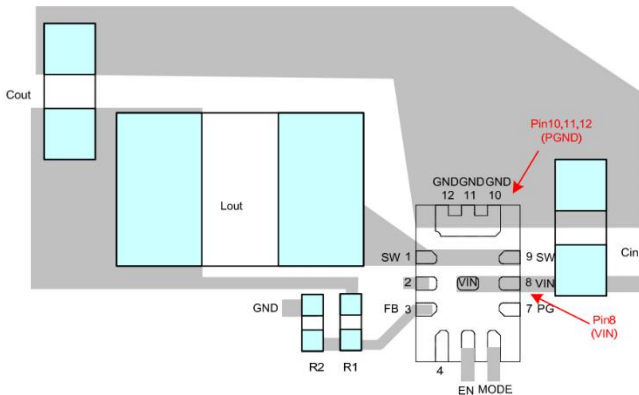
图 35. GM25002 PCB 推荐布局
