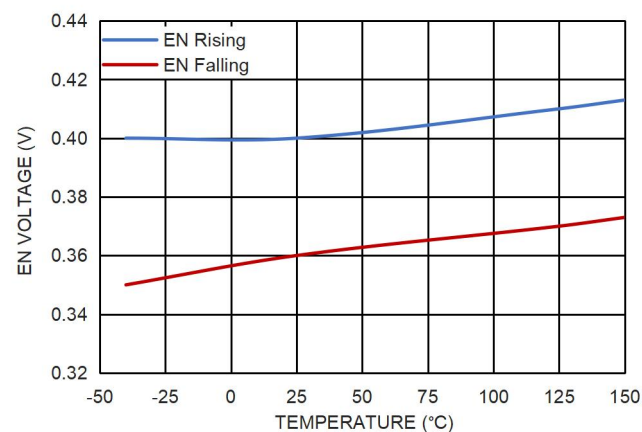
图 23. EN 阈值和温度的关系
