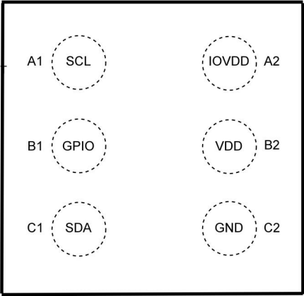
引脚功能
