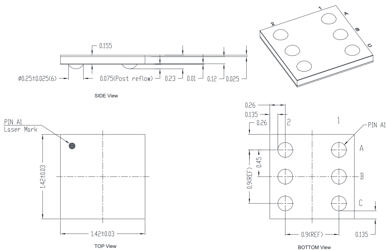
WLCSP-6
