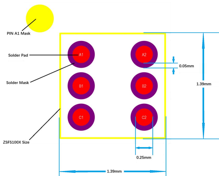
图 12 ZSFS1001 封装焊盘图
