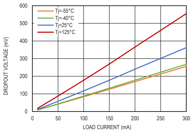
图 8. 7.0V 压差电压和负载电流的关系
