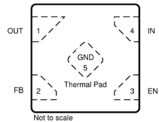
图 4.5 引脚 DFN-5 引脚配置（可调输出，顶视图）
