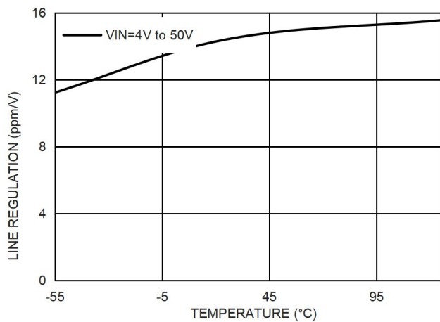
图 13. 输入调整率和温度的关系, V_{OUT}=2.5V
