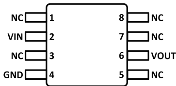
图 3. TSSOP-8 引脚配置(顶视图)
