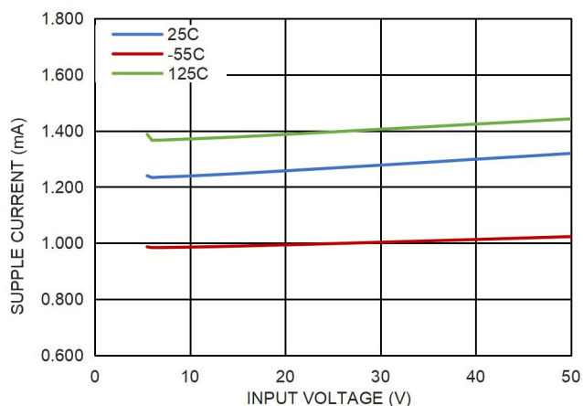
图 19. 输入电流和输入电压的关系, V_{OUT}=5.0V
