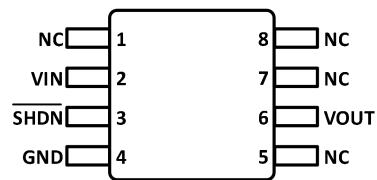
图 3. MSOP-8 引脚配置(顶视图)
