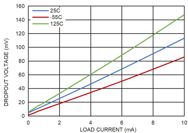
图 23.最小输入电压和输出电压的关系, V_{OUT}=5.0V
