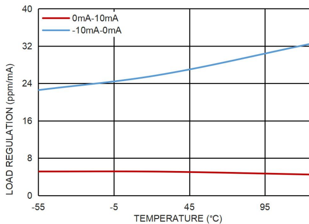
图 11. 负载调整率和温度的关系, V_{OUT}=5.0V
