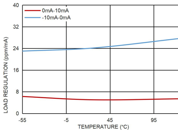
图 12. 负载调整率和温度的关系, V_{OUT}=10.0V
