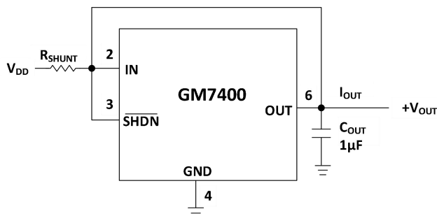
图 27. 正压并联方式
