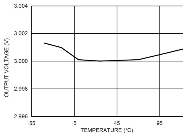
图 6. 3.0V 输出电压和温度的关系
