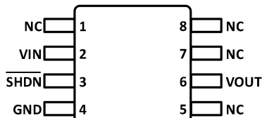
图 1. 8 引脚 MSOP
