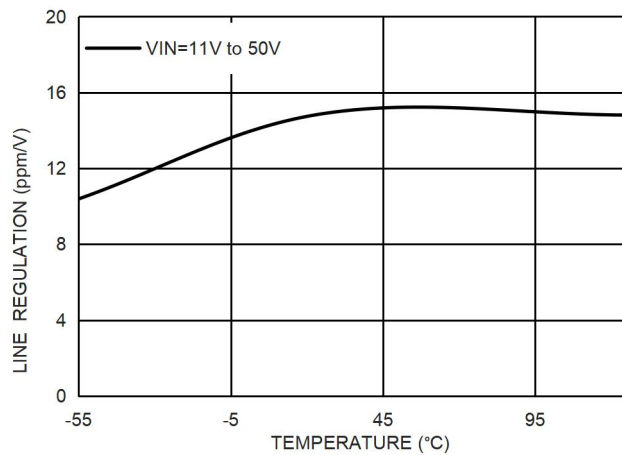
图 16. 输入调整率和温度的关系, V_{OUT}=10.0V
