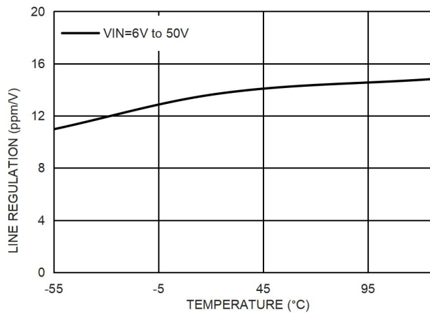
图 15. 输入调整率和温度的关系, V_{OUT}=5.0V
