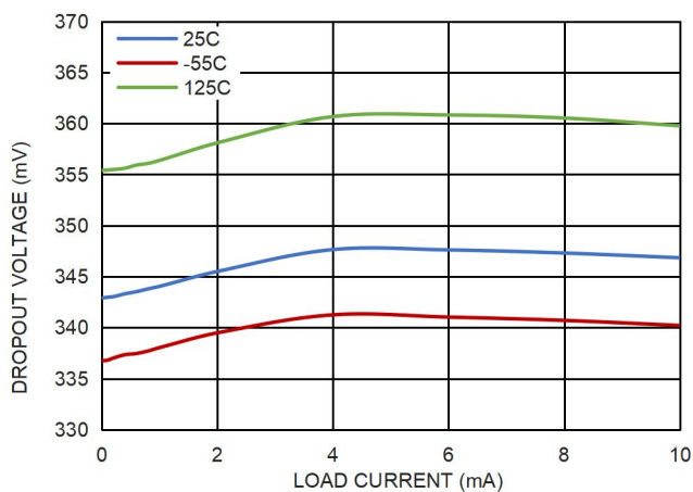
图 21. 最小输入电压和输出电压的关系, V_{OUT}=2.5V
