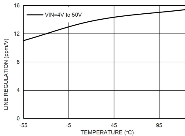
图 14. 输入调整率和温度的关系, V_{OUT}=3.0V
