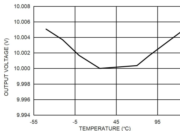
图 8. 10.0V 输出电压和温度的关系
