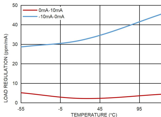
图 10. 负载调整率和温度的关系, V_{OUT}=3.0V
