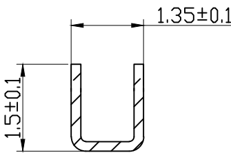
C-C
