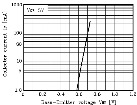
Fig. 2 I_C - V_{BE}
