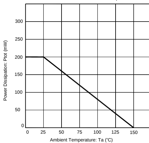
Fig. 6 P_{tot} - T_a
