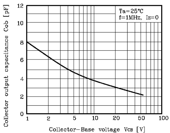
Fig. 5 C_{ob} - V_{CB}
