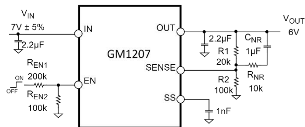
图 30. 噪声优化
