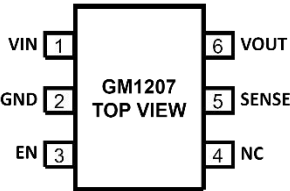
图 5.6 引脚 SOT-23 引脚配置
