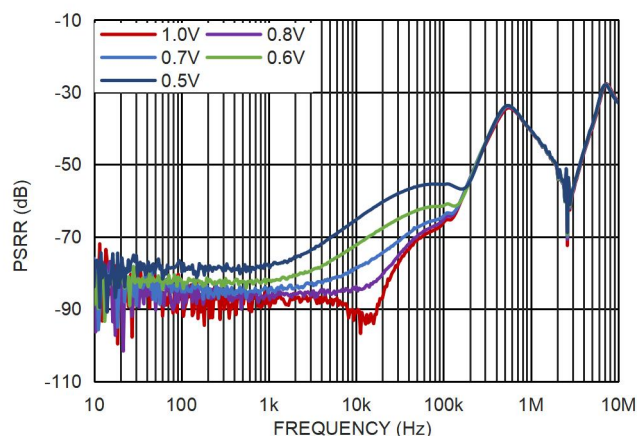
图 20. 电源电压纹波抑制比与压差的关系, V_{OUT}=5.0V
