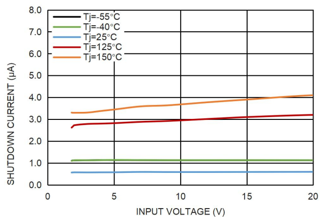
图 10. 关机电流和输入电压的关系
