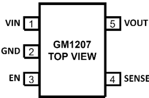
图 4.3 引脚 SOT-23 引脚配置
