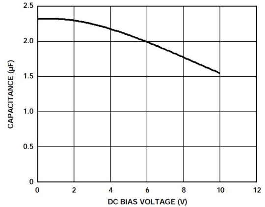
图 27. 电容与电压关系特性
