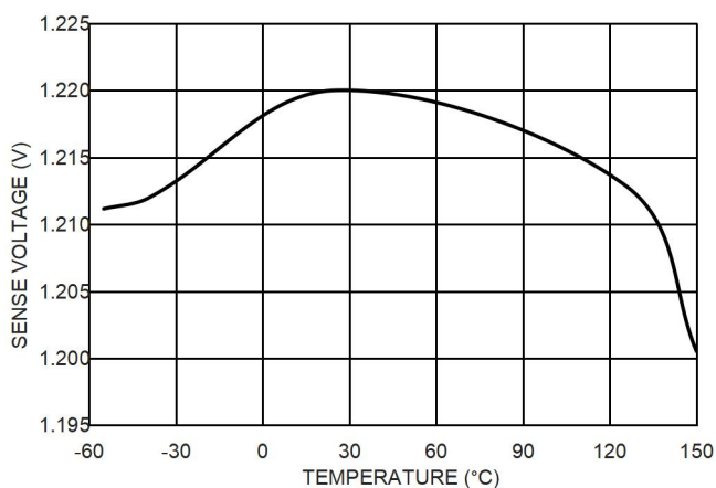
图 15. 1.22V SENSE 引脚电压精度
