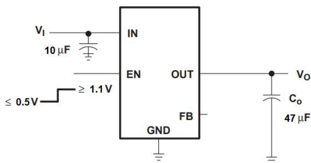
图 1 GM12033 典型应用
