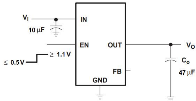
图 6 固定输出电压
