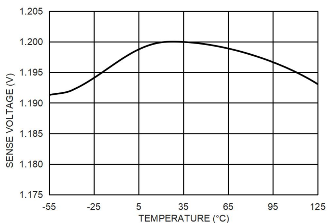
图 13. 1.2V SENSE 引脚电压精度
