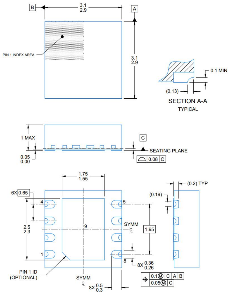
图 30.8 引脚 DFN, 3mm x 3mm
