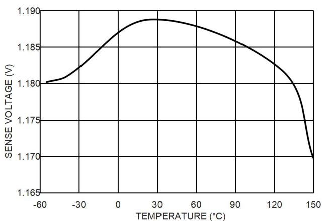
图 14. 1.18V SENSE 引脚电压精度
