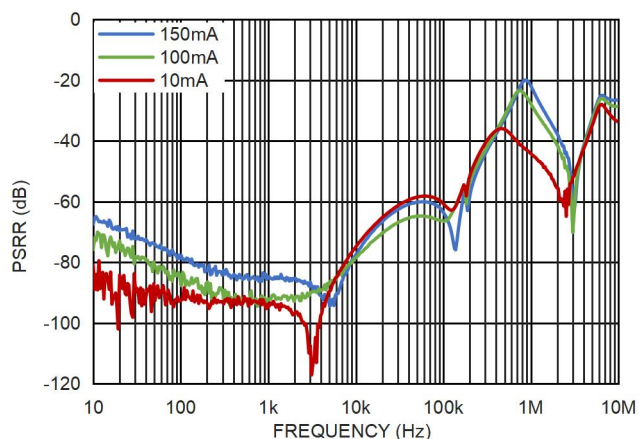
图 21. 电源电压纹波抑制比与负载的关系, V_{OUT}=5.0V
