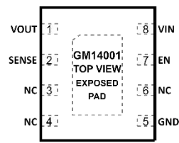
图 3. 8 引脚 DFN 的引脚配置
