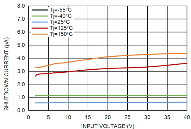
图 9. 关机电流和输入电压的关系
