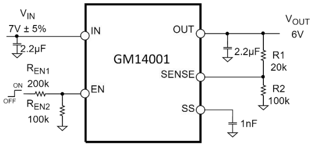
图 28. EN 引脚的典型分压器
