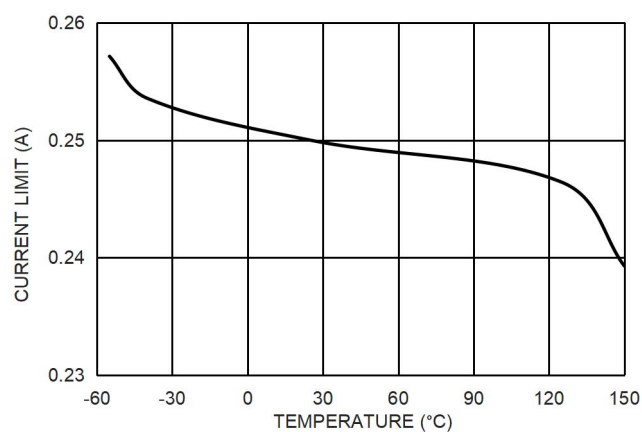
图 15. 输出限流值和温度的关系
