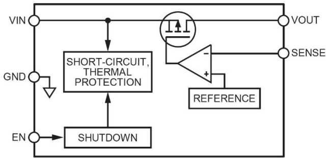
图 24. 内部框图
