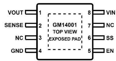
图 5. 8 引脚 MSOP 的引脚配置
