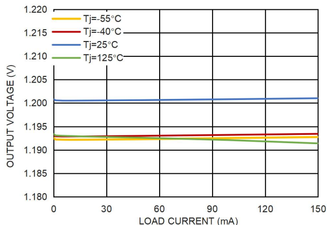
图 10. 1.2V 输出电压和负载电流的关系
