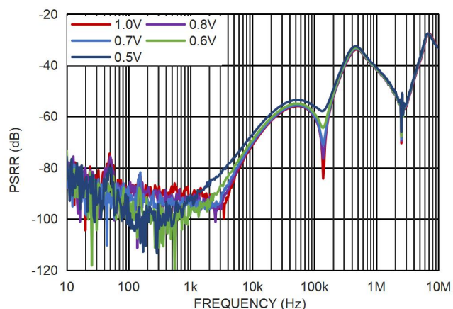
图 19. 电源电压纹波抑制比与压差的关系, V_{OUT}=5.0V
