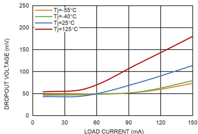
图 7. 5.0V 压差电压和负载电流的关系
