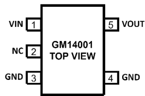
图 4. 5 引脚 SOT 引脚配置
