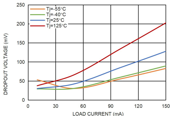
图 6. 3.3V 压差电压和负载电流的关系
