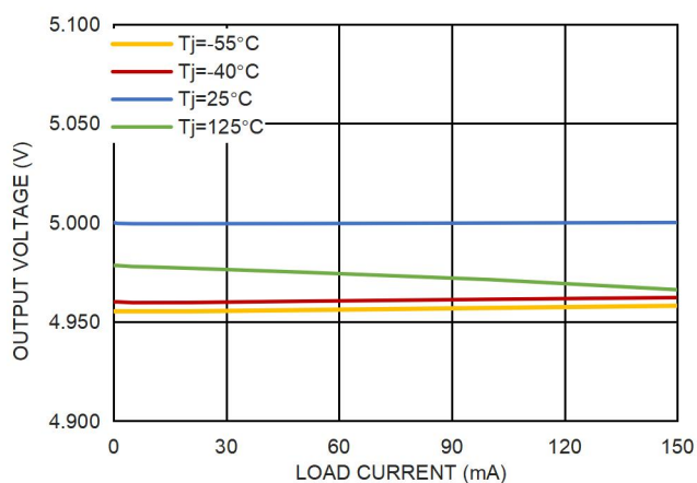
图 12. 5.0V 输出电压和负载电流的关系
