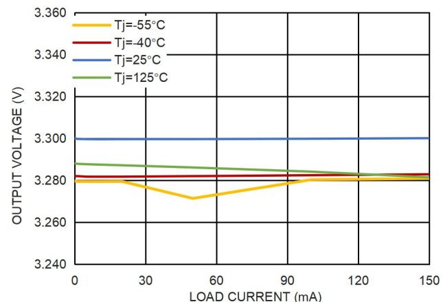
图 11. 3.3V 输出电压和负载电流的关系
