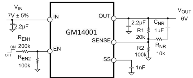
图 29. 噪声优化
