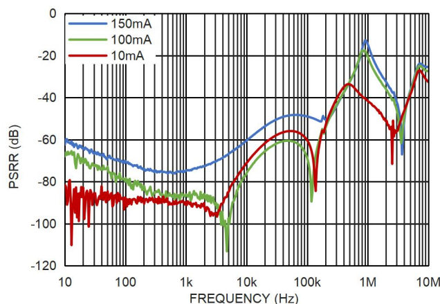
图 20. 电源电压纹波抑制比与负载的关系, V_{OUT}=3.3V
