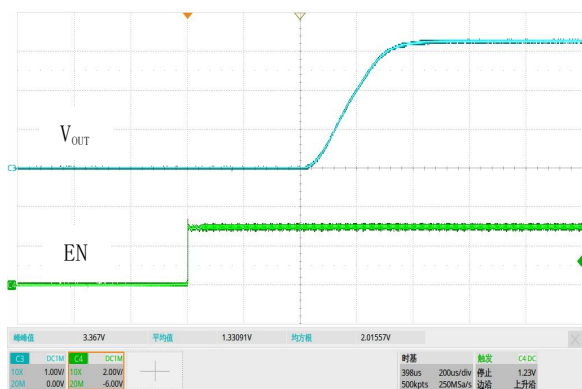
图 22. 软启动, V_{IN}=4.3V , V_{OUT}=3.3V , I_{OUT}=150mA
