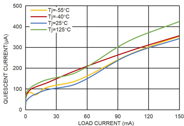
图 8. 静态电流和负载电流的关系, V_{IN} = 4.3V
