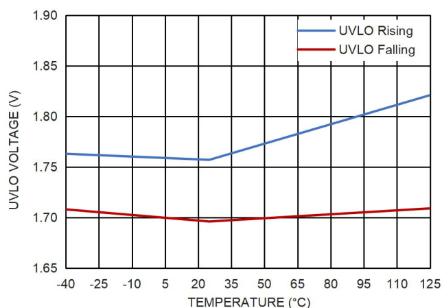
图 14. UVLO 阈值
