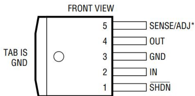
图 3 引脚配置
