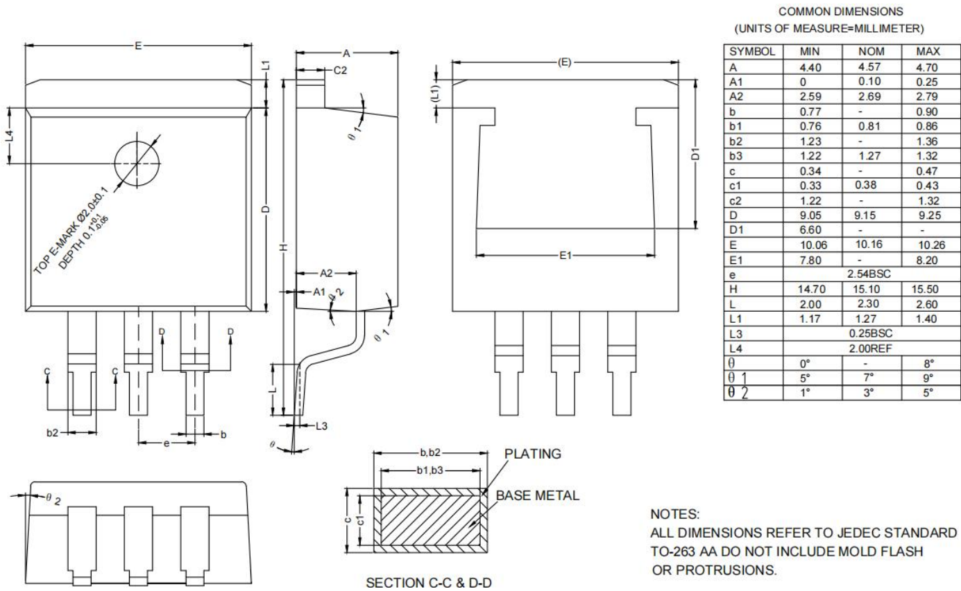
图 21. 3 引脚 TO-263
