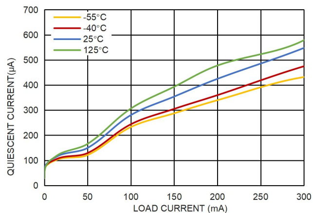
图 10. 静态电流和负载电流的关系, V_{IN}=4.3V
