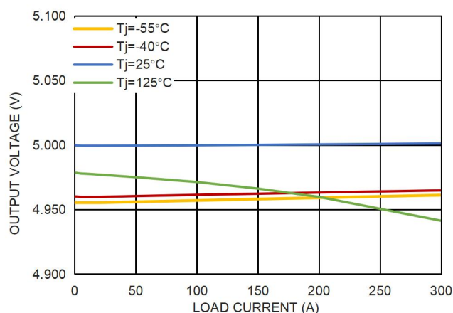
图 14. 5.0V 输出电压和负载电流的关系
