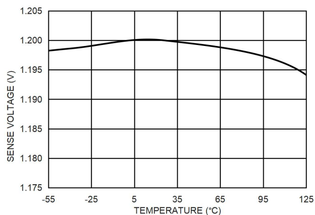
图 15. 1.2V SENSE 引脚电压精度
