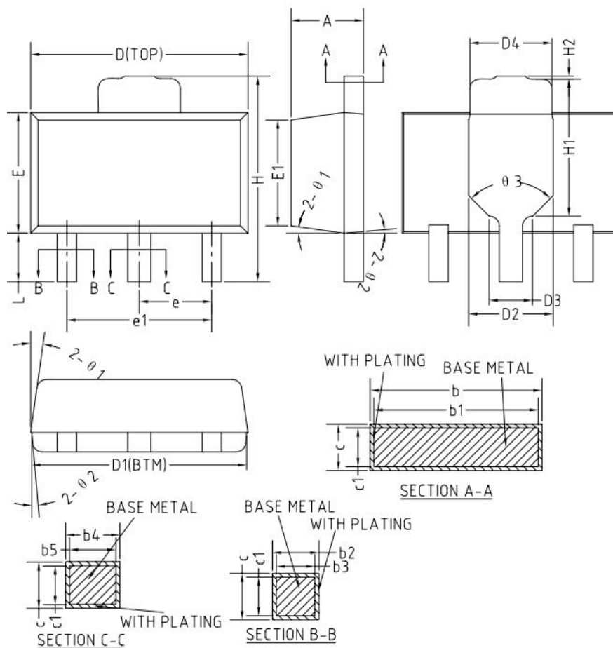
图 37.3 引脚 SOT-89
