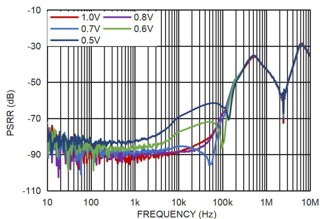
图 20. 电源电压纹波抑制比与压差的关系, V_{OUT}=3.3V
