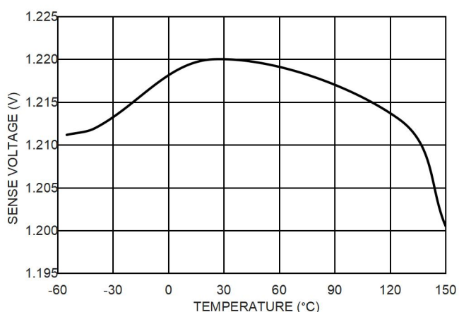
图 16. 1.22V SENSE 引脚电压精度
