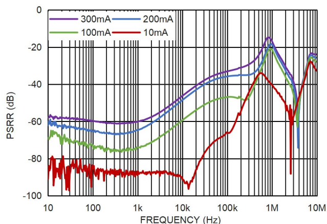
图 23. 电源电压纹波抑制比与负载的关系, V_{OUT}=5.0V
