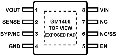
图 5.8 引脚 DFN 的引脚配置
