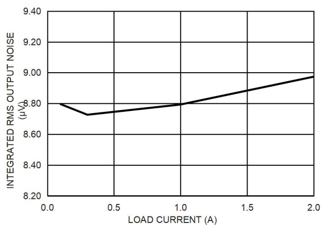
图 15. 积分 RMS 输出噪声, V_{IN}=5V , V_{OUT}=3.3V
