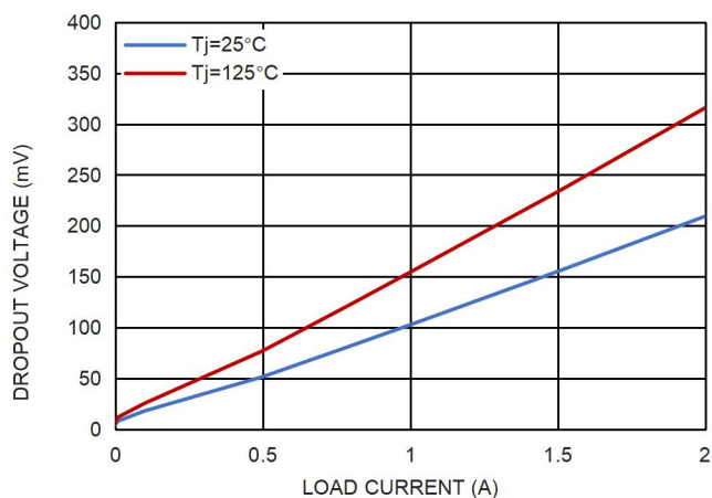
图 3. 压差电压和负载电流的关系
