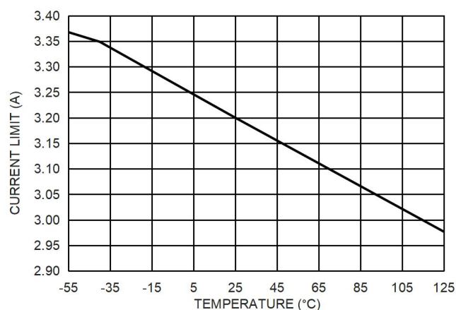
图 11. 输出限流值和温度的关系
