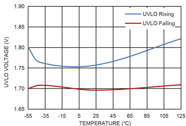
图 13. UVLO 阈值
