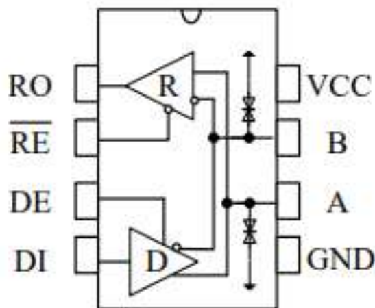
图 1 SN65HVD11DR (ES) 引脚分布图
