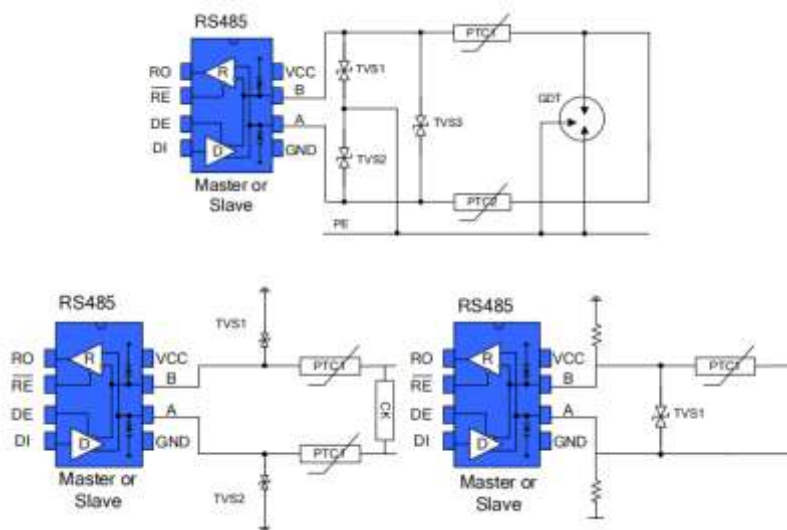
图 11 端口防护方案
