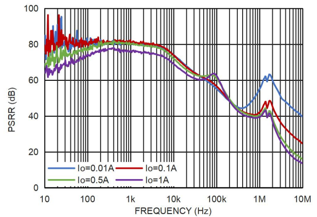
图 20. 电源电压纹波抑制比, V_{IN}=5V , V_{OUT}=3.3V
