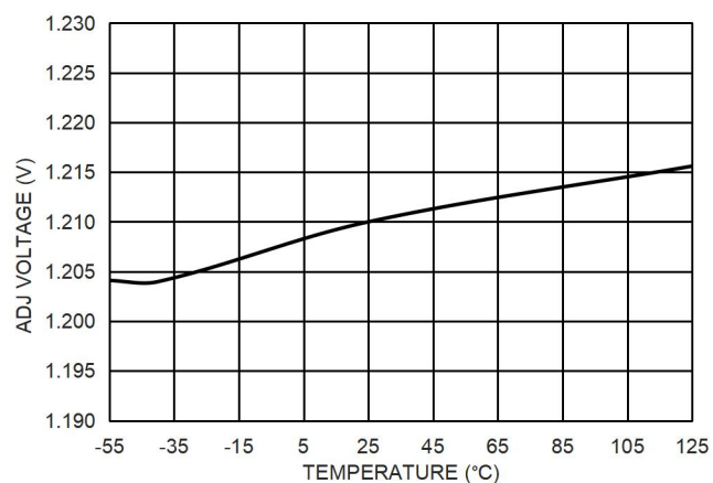
图 14. ADJ 引脚电压精度
