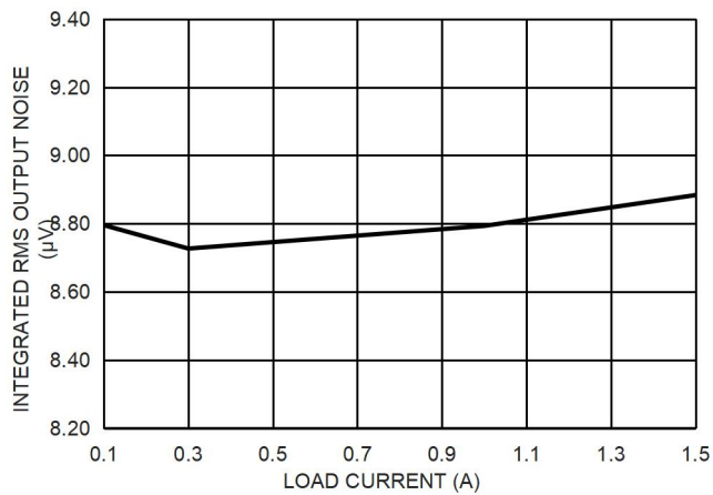
图 19. 积分 RMS 输出噪声, V_{IN}=5V , V_{OUT}=3.3V
