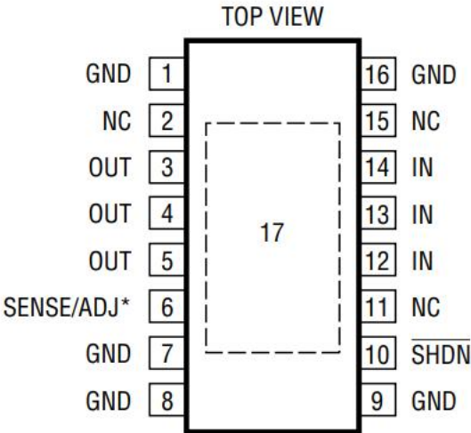
16 引脚 TSSOP 裸露焊盘必须焊接到 PCB 上 图 5 引脚配置
