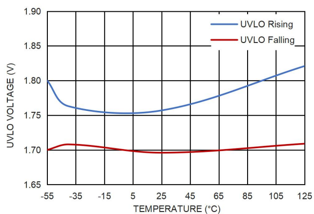
图 17. UVLO 阈值
