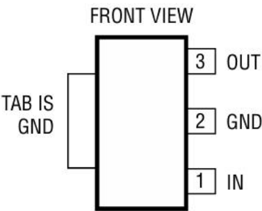
3 引脚 SOT-223 裸露焊盘必须焊接到 PCB 上 图 6 引脚配置
