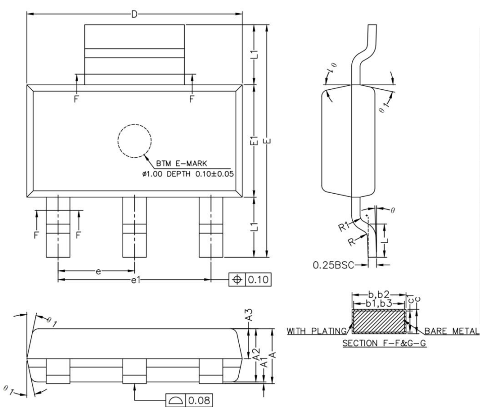
图 27.3 引脚 SOT-223
