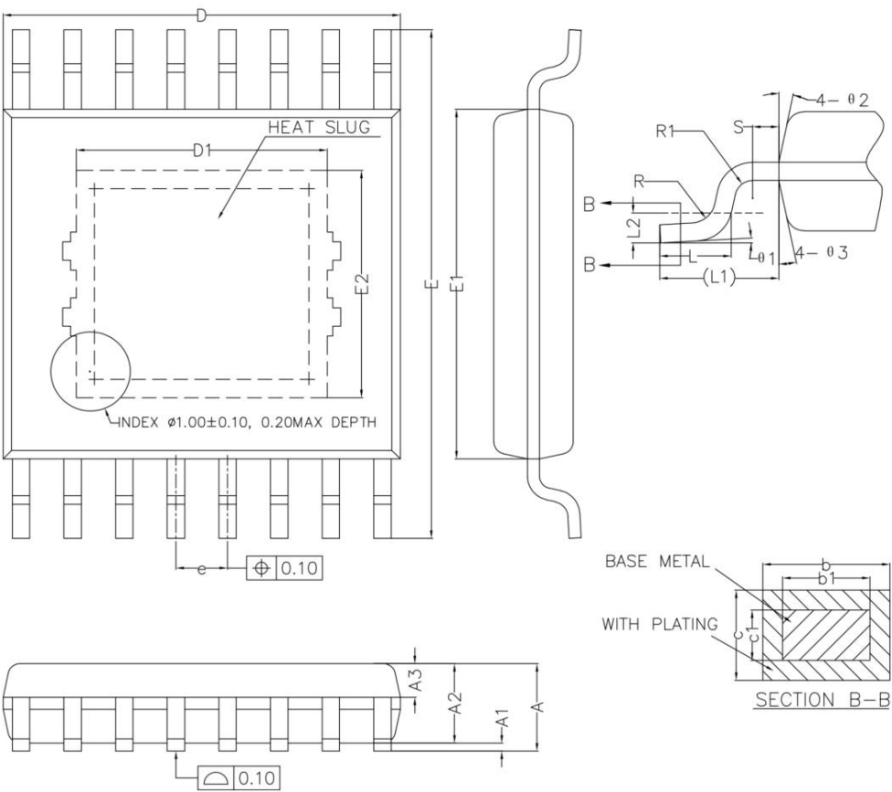
图 26.16 引脚 TSSOP
