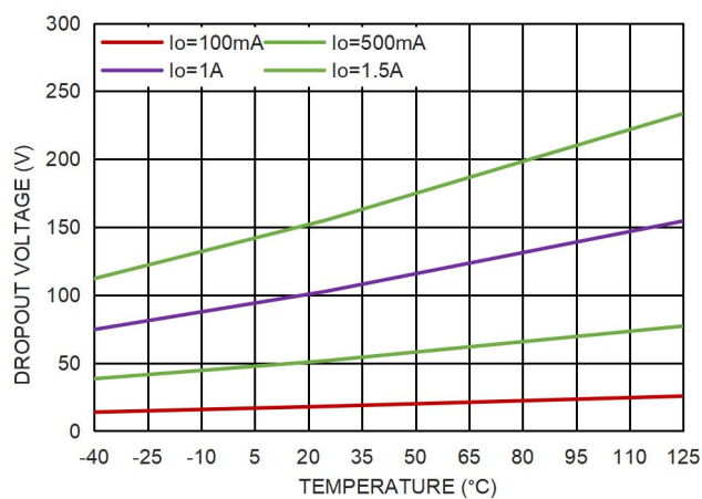
图 8. 压差电压和温度的关系
