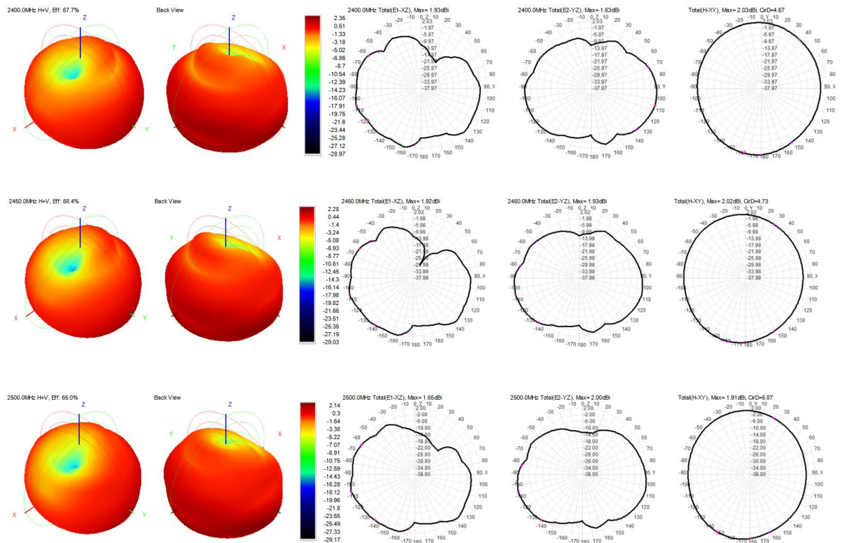
图 10 天线场型图
