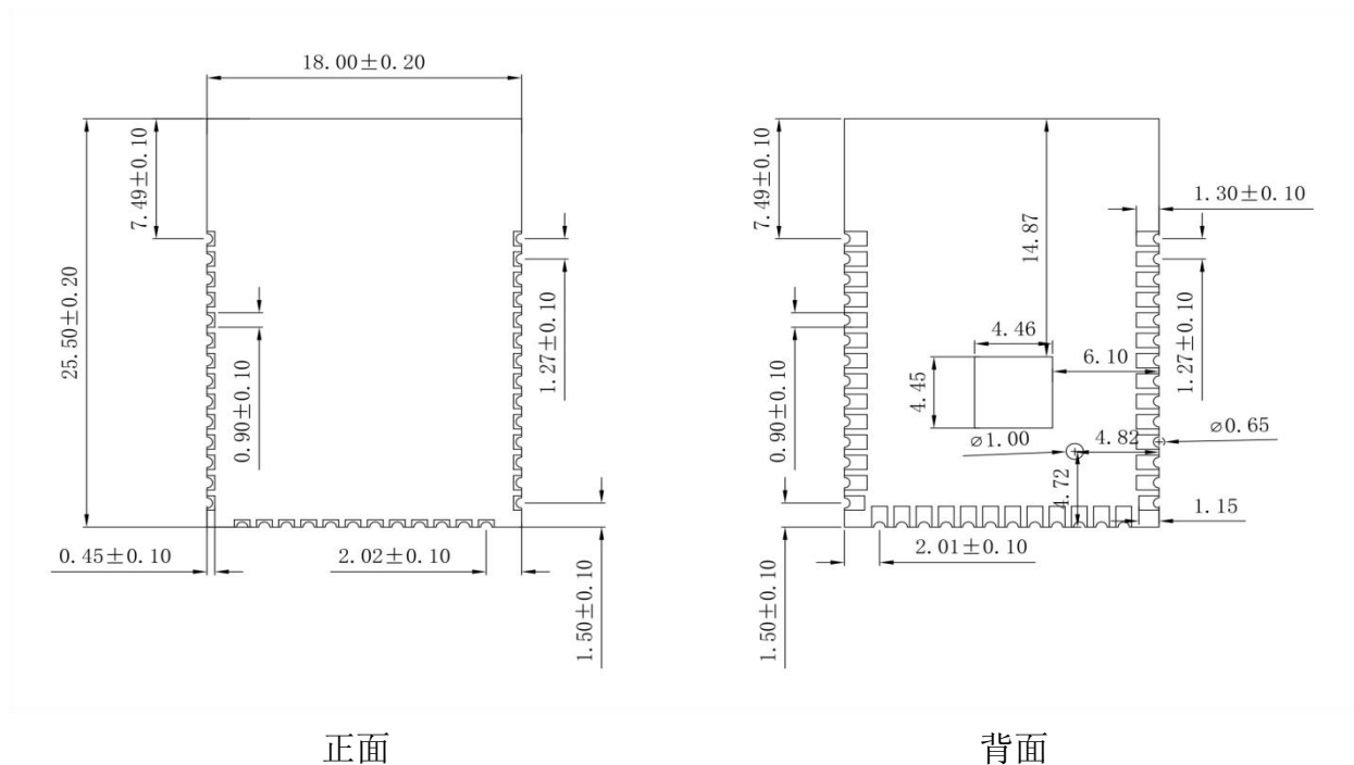
图 4 尺寸图
