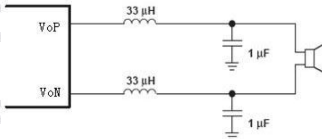
输出加 LC 滤波器典型应用电路
