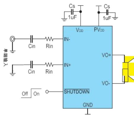
图2 WT8302单端输入方式应用图
