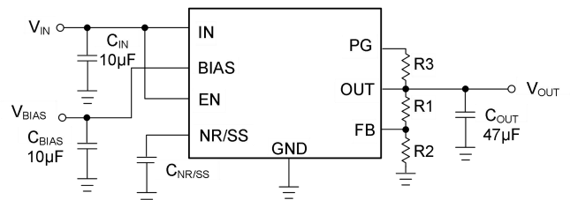
图 1. GM1203-1 典型应用
