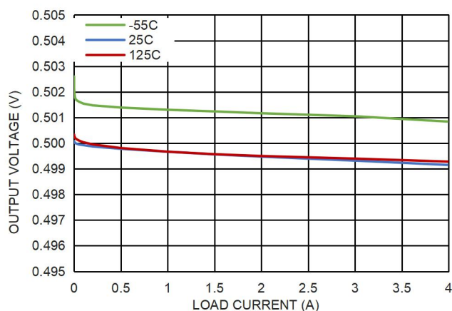
图 9. 负载调整率, BIAS 浮空
