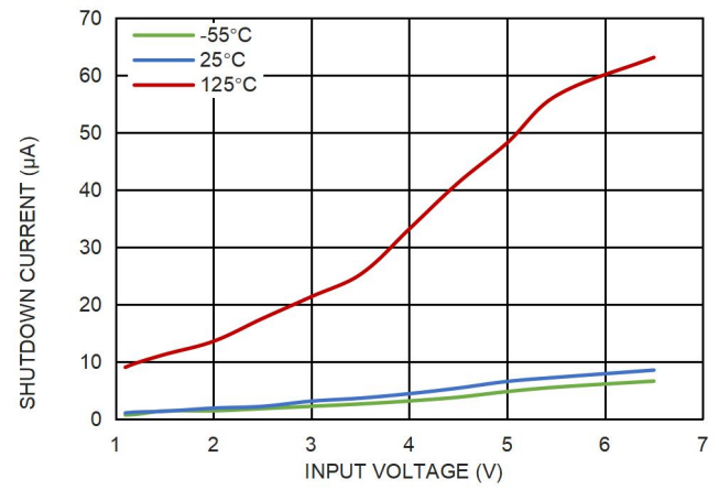
图 15. 停机静态电流和输入电压的关系
