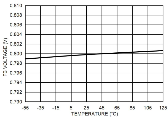
图 26. FB 引脚电压和温度的关系
