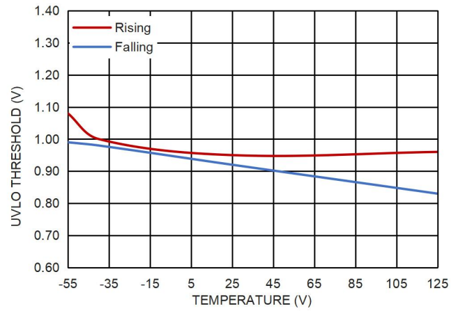
图 17. UVLO 阈值, V_{BIAS} = 5V
