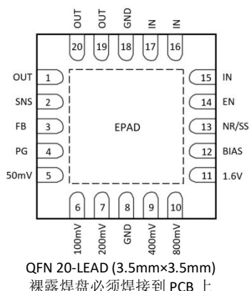
图 6 引脚配置
