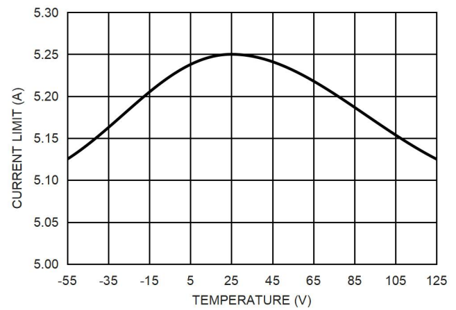
图 19. GM1203-3 输出限流值和温度的关系
