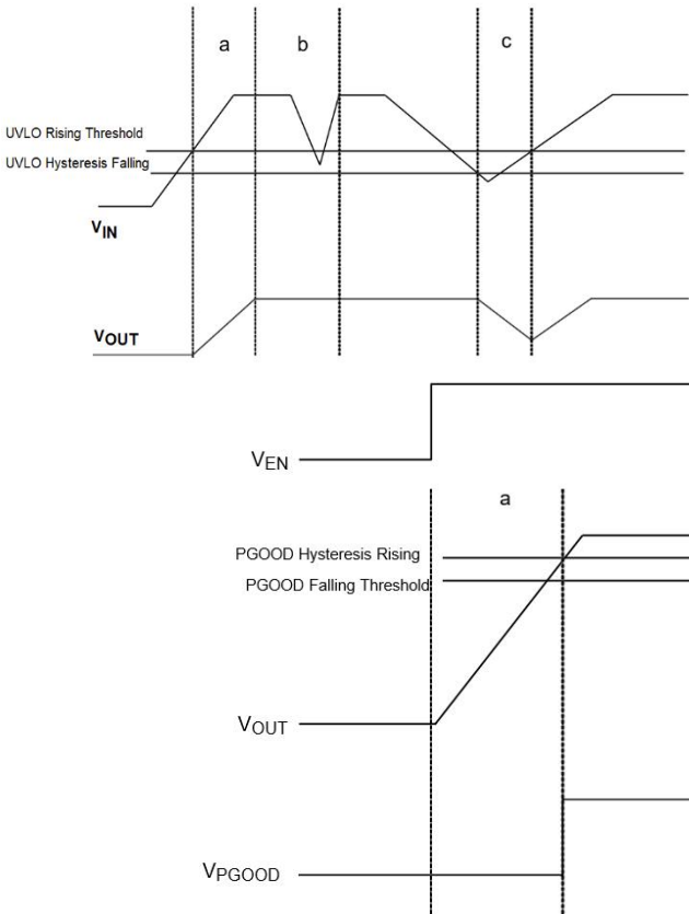
图 32 .PG 触发场景具有不同的运行状态
