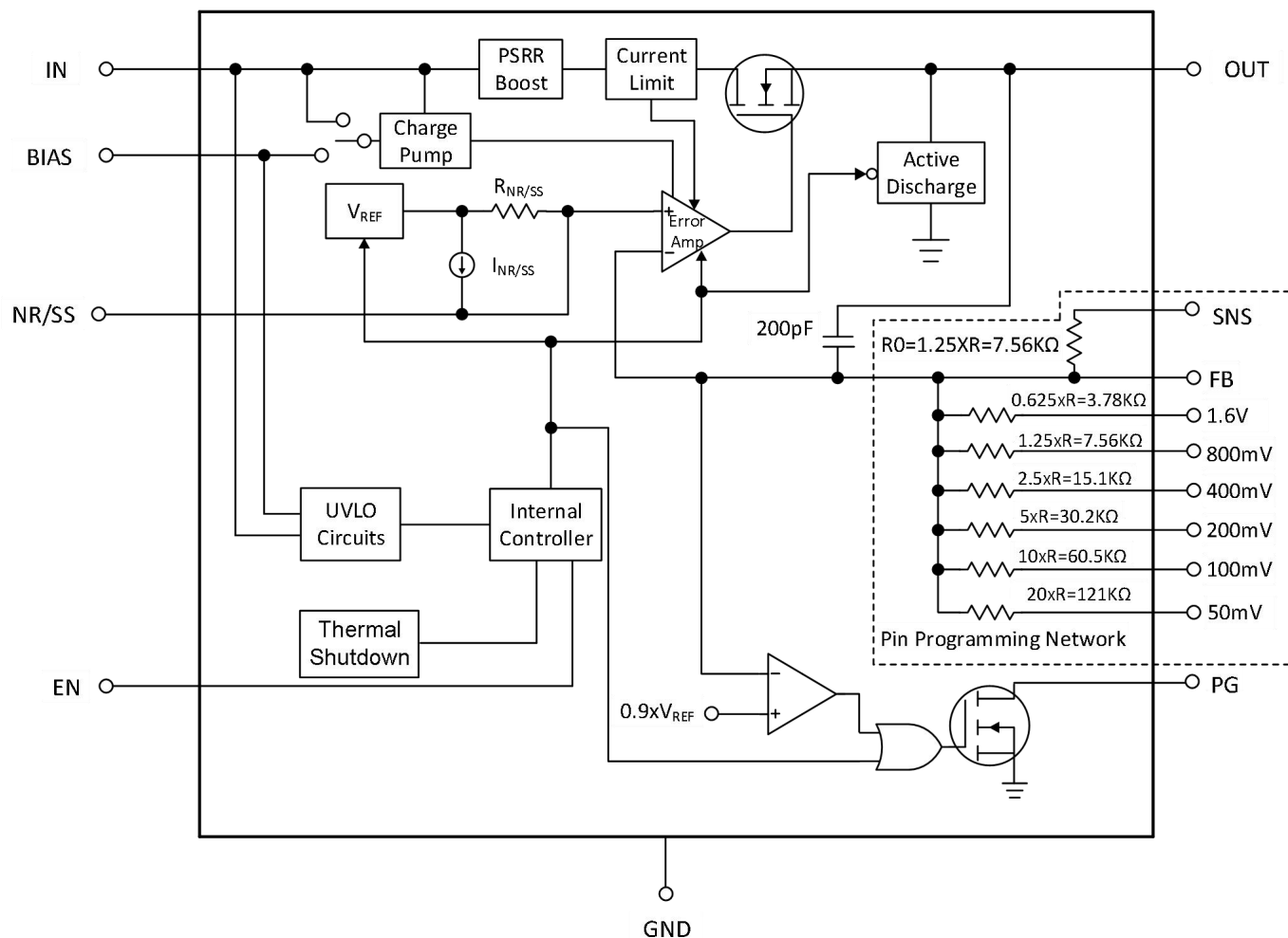
图 4. GM1203B-1 方框图
