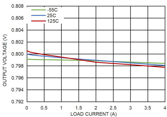
图 28. 负载调整率, V_{BIAS} = 5V
