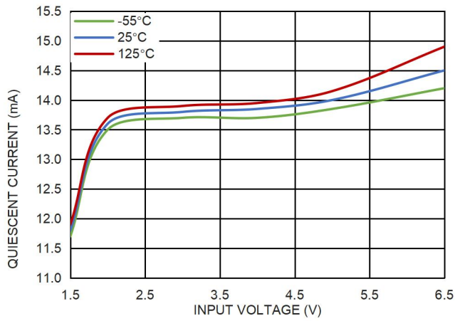
图 14. 静态电流和输入电压的关系, I_{OUT}=1mA
