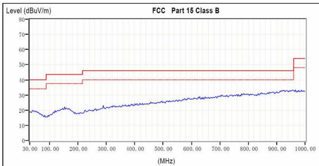
EMI 测试频谱图
