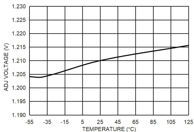
图 11. ADJ 引脚电压精度
