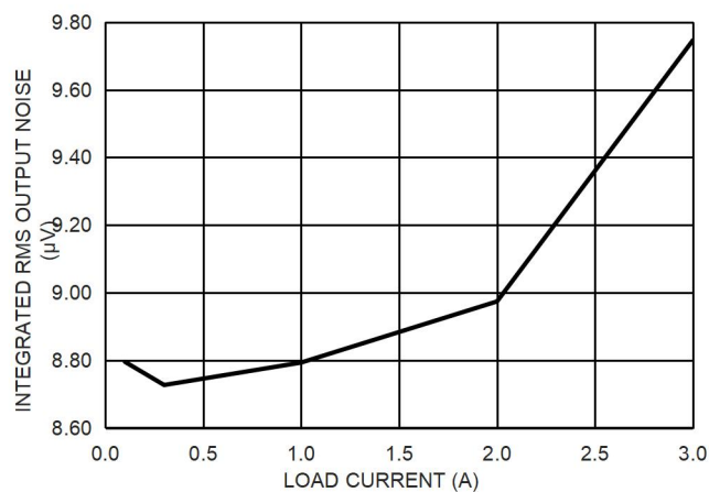
图 16. 积分 RMS 输出噪声, V_{IN}=5V , V_{OUT}=3.3V
