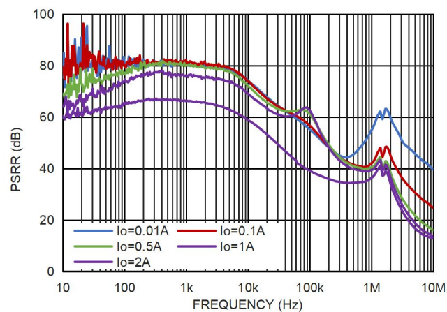
图 17. 电源电压纹波抑制比, V_{IN}=5V , V_{OUT}=3.3V
