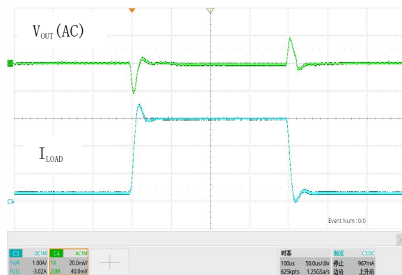
图 19. 负载瞬态响应, V_{IN}=2.8V , V_{OUT}=1.8V , I_{OUT}=0.3A to 3A
