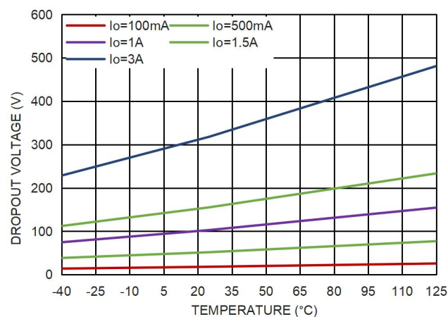
图 5. 压差电压和温度的关系
