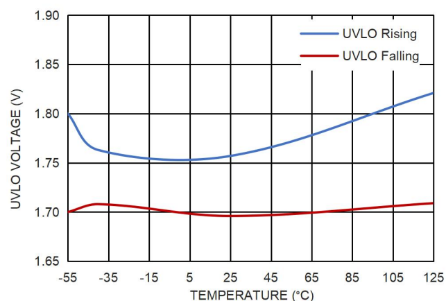
图 14. UVLO 阈值
