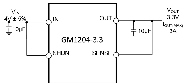
图 1 典型应用
