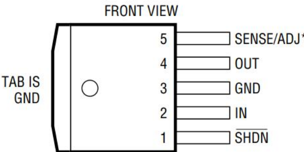
5 引脚 TO-263 裸露焊盘必须焊接到 PCB 上
