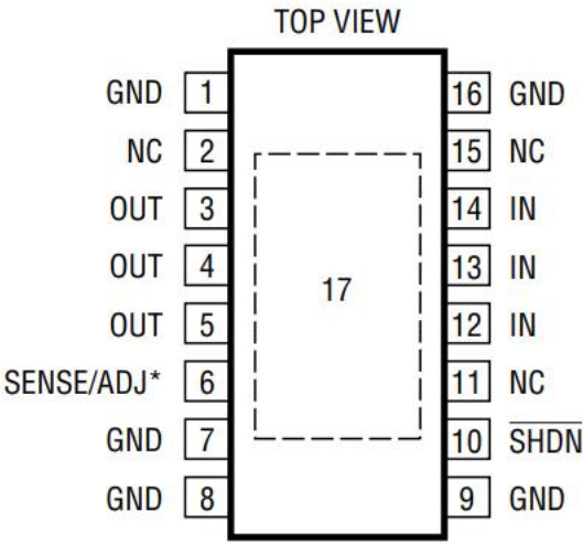
16 引脚 TSSOP 裸露焊盘必须焊接到 PCB 上 图 3 引脚配置
