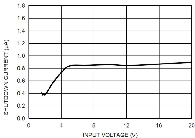
图 7. 关机电流和输入电压的关系
