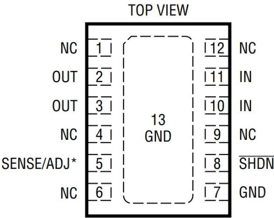
12 引脚 DFN 裸露焊盘必须焊接到 PCB 上 图 3 引脚配置
