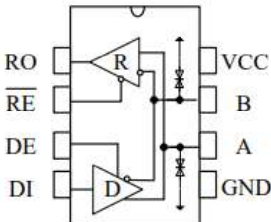
图 1 SN65HVD3088EDR (ES) 引脚分布图
