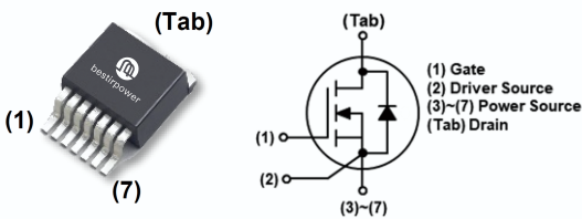
TO-263-7L
