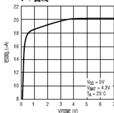
弱下拉状态下的 \overline{\text{CHRG}} 引脚 I-V 曲线
