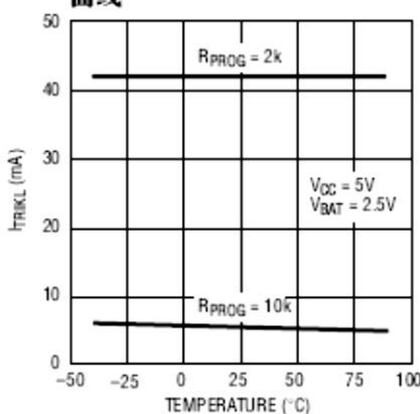
涓流充电电流与温度的关系曲线
