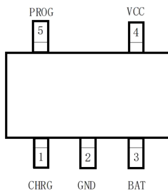
SOT-23-5
