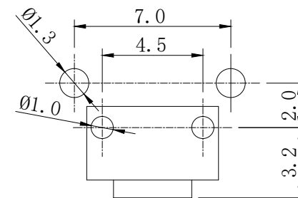
PCB线路板安装图( \pm 0.1 )
