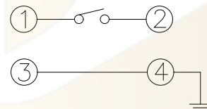
电路图
