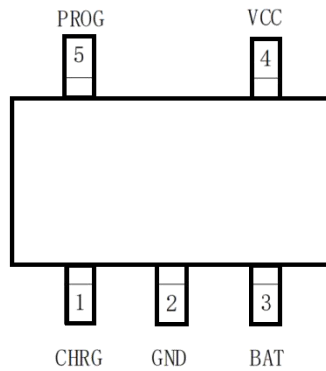
SOT-23-5
