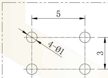
PCB线路板安装图(±0.1)
