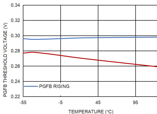
图 20. PGFB pin 阈值
