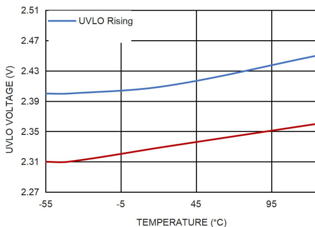
图 17. UVLO 阈值
