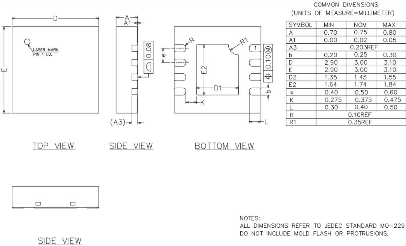
图 33. DFN-8 封装 (3mmx3mm)
