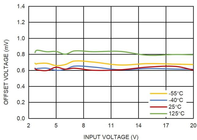
图 10. |V_{OUT} - V_{SET}| 和输入电压的关系, V_{OUT} = 1.8V
