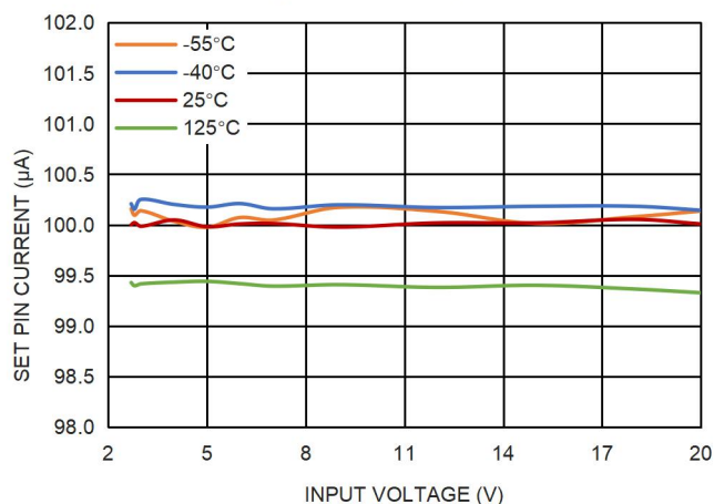
图 8. SET pin 电流和输入电压的关系
