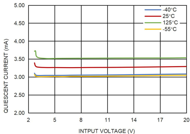
图 14. 静态电流和输入电压的关系, I_{OUT}=10mA
