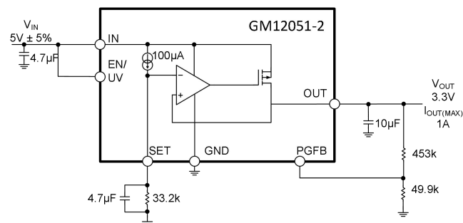
图 1 典型应用
