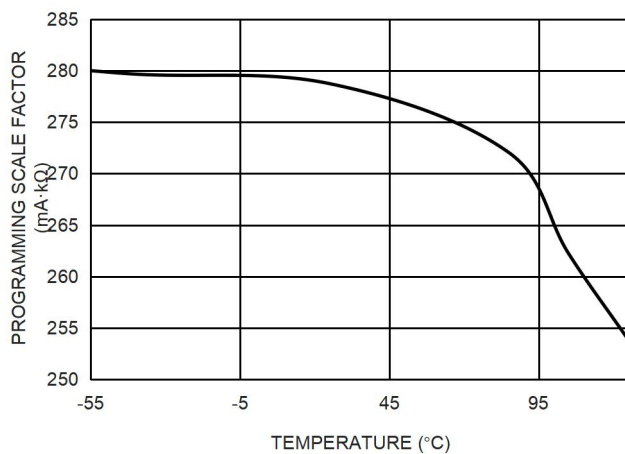
图 19. 输出限流值编程因子
