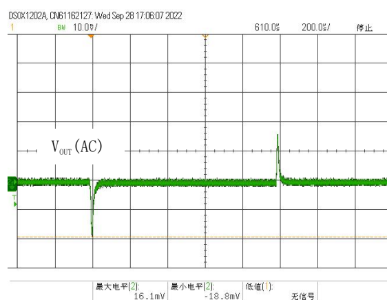
图 25. 负载瞬态响应, V_{IN}=4.3V , V_{OUT}=3.3V , I_{OUT}=1mA to 1A
