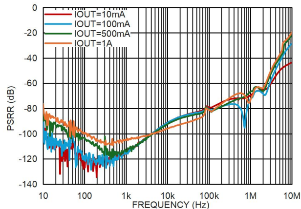
图 23. 电源电压纹波抑制比, V_{IN}=5V , V_{OUT}=3.3V
