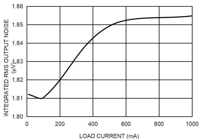
图 22. 积分 RMS 输出噪声, V_{IN}=5V , V_{OUT}=3.3V
