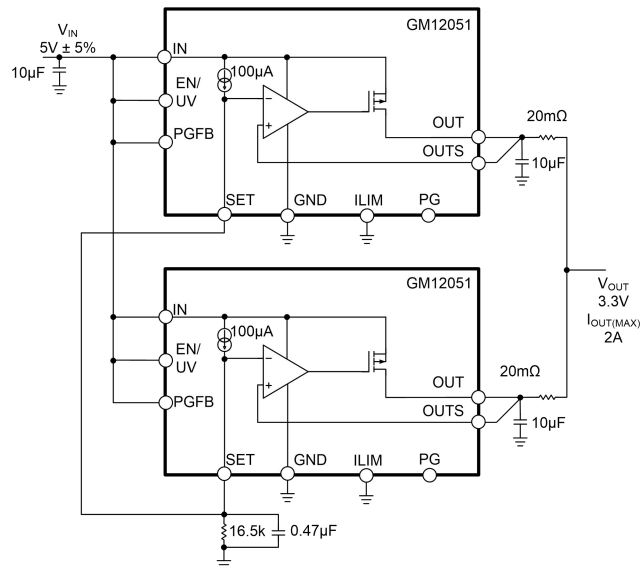
图 28. 并联设备
