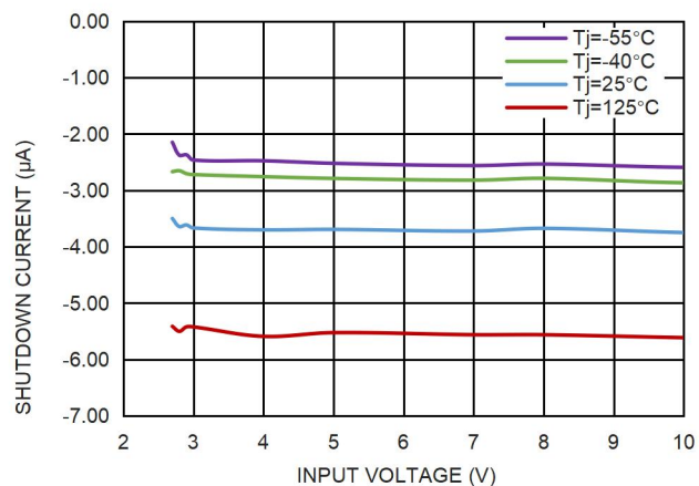
图 8. 静态电流与输入电压的关系
