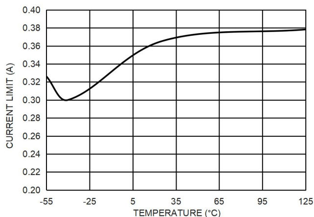
图 15. 限流值和结温的关系
