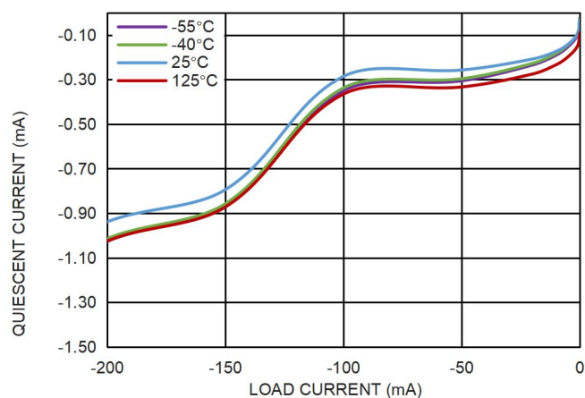
图 7. 静态电流与负载电流的关系
