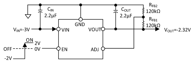
图 1 典型应用
