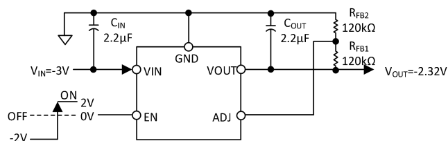
图 20. 设置可调输出电压
