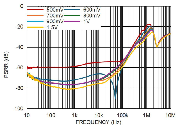
图 11. PSRR 和压差的关系, I_o = 200\text{mA}
