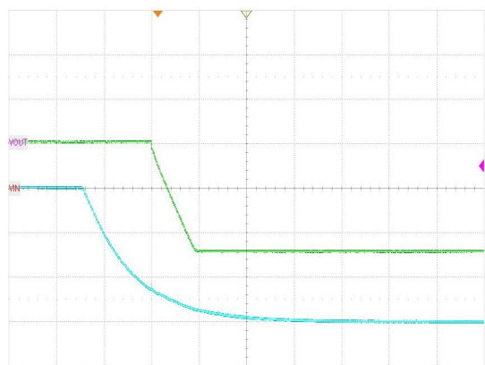
图 16. 软启动, V_{IN} = -6V , V_{OUT} = -5V , I_O = -200mA
