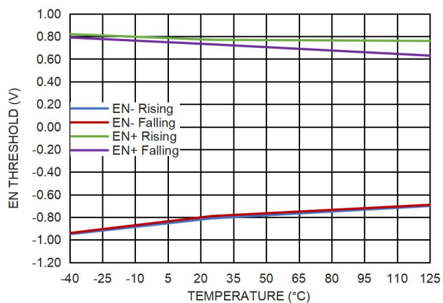
图 14. EN 阈值和结温的关系
