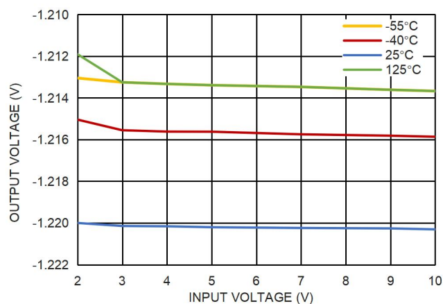
图 6. ADJ 引脚电压与 vs. 输入电压的关系
