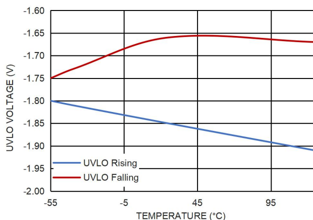
图 13. UVLO 阈值和结温的关系
