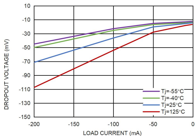
图 9. 压差电压和负载电流的关系
