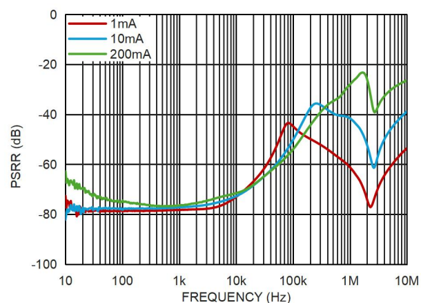
图 12. PSRR 和负载电流的关系
