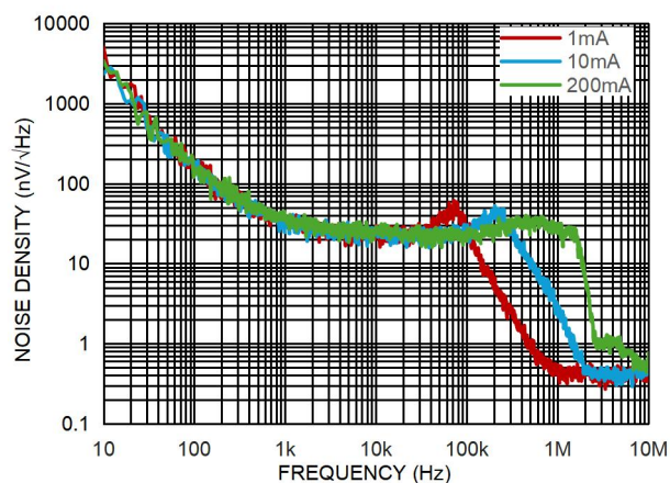
图 10. 噪声谱密度
