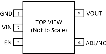
图 2. SOT-23 引脚配置(顶视图)
