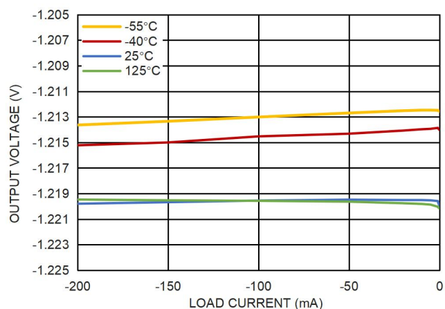
图 5. ADJ 引脚电压与 vs. 负载电流的关系
