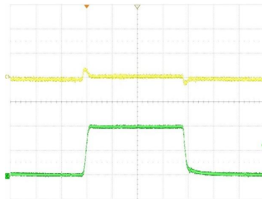
图 17. 负载瞬态响应, V_{IN} = -6V , V_{OUT} = -5V , I_O = -10 至-200mA
