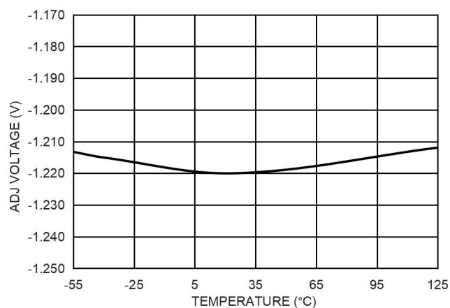
图 4. ADJ 引脚电压与结温 (Tj) 的关系
