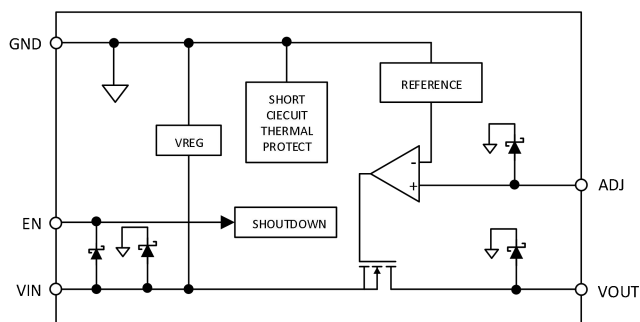
图 19. 可选输出电压型号内部框图
