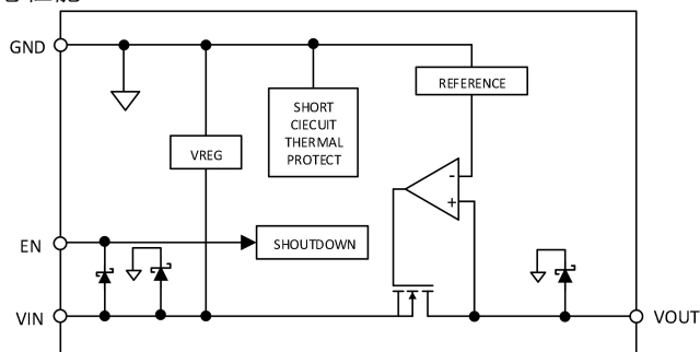
图 18. 固定输出电压内部框图
