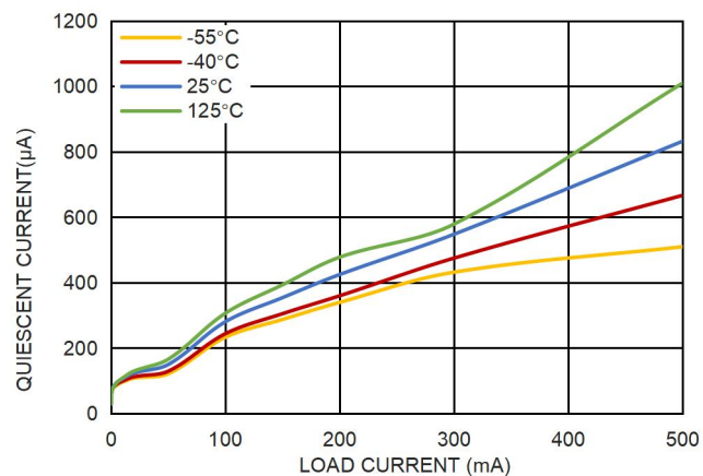
图 9. 静态电流和负载电流的关系, V_{IN}=4.3\text{V}
