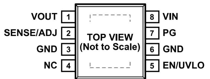
图 6.8 引脚 SOP-8 的引脚配置
