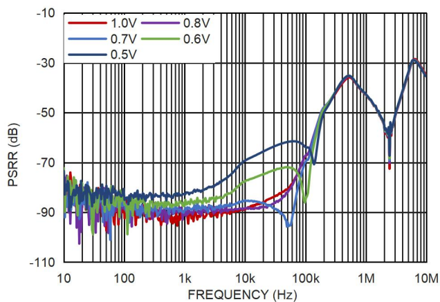
图 19. 电源电压纹波抑制比与压差的关系, V_{OUT}=3.3V
