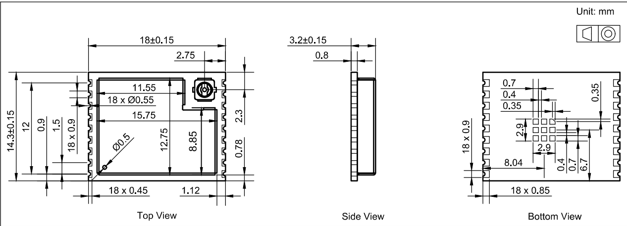
图 10-2. ESP32-C3-WROOM-02U 尺寸
