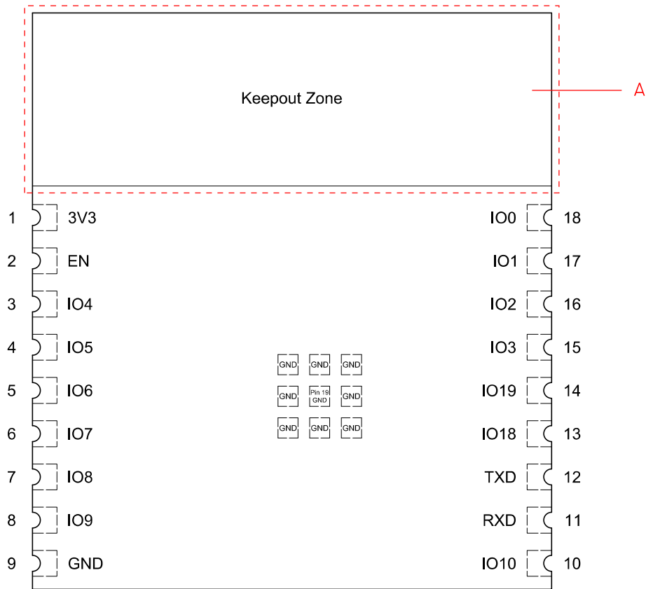
图 3-1. 管脚布局（顶视图）
