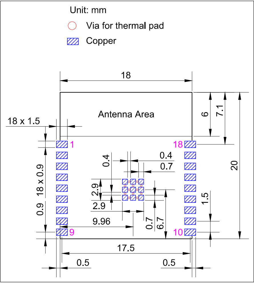
图 11-1. ESP32-C3-WROOM-02 推荐 PCB 封装图形
