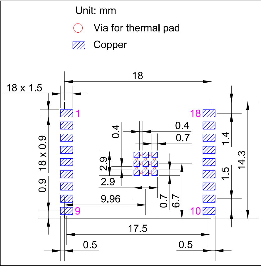
图 11-2. ESP32-C3-WROOM-02U 推荐 PCB 封装图形
