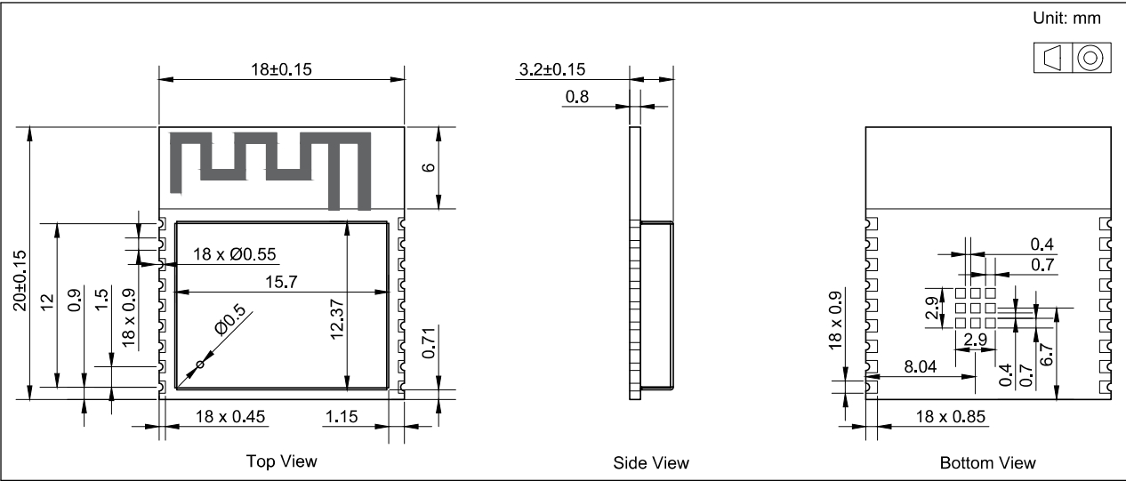
图 10-1. ESP32-C3-WROOM-02 尺寸
