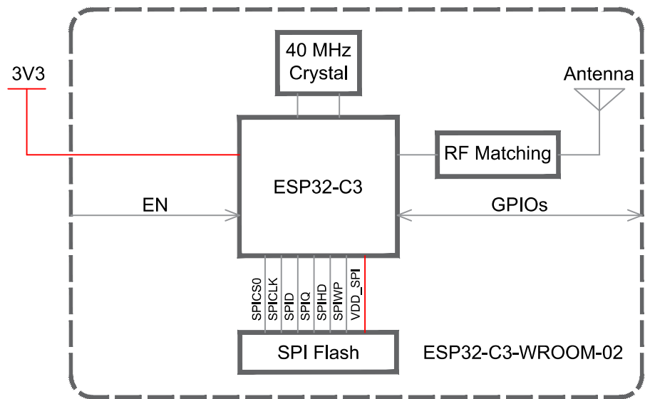
图 2-1. ESP32-C3-WROOM-02 功能框图
