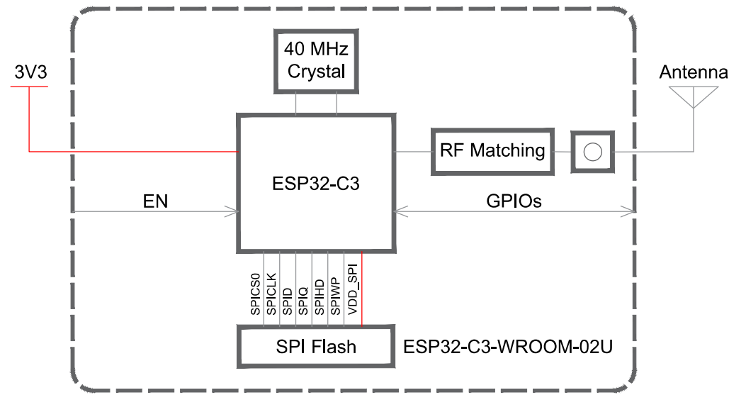
图 2-2. ESP32-C3-WROOM-02U 功能框图
