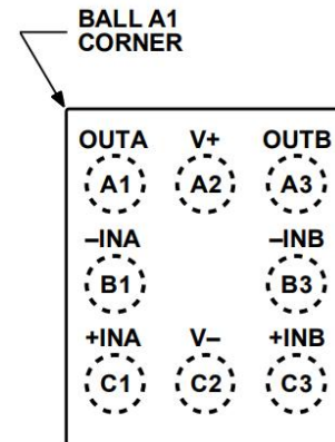
图 2. 8-Ball WLCSP
