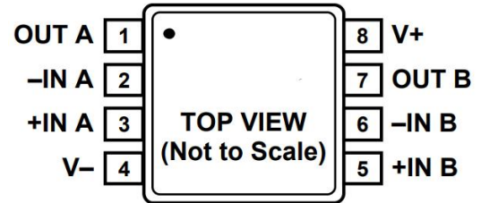
图 1. 8 引脚 MSOP 和 SOP
