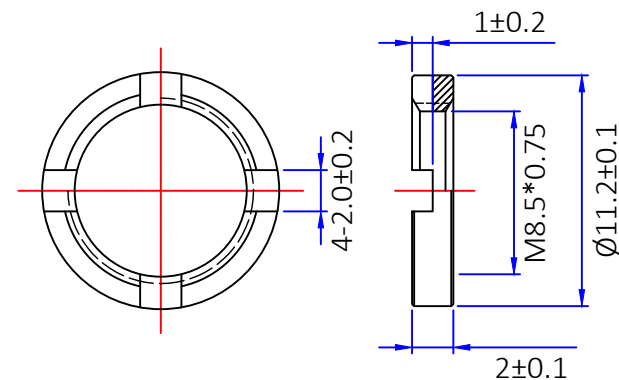
圆形螺母
