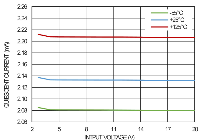
图 10. 静态电流和输入电压的关系, I_{OUT}=10mA
