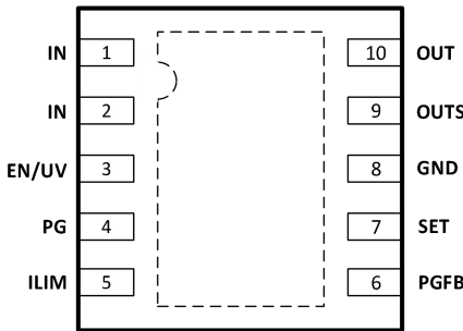
图 2. DFN 引脚配置(顶视图)
