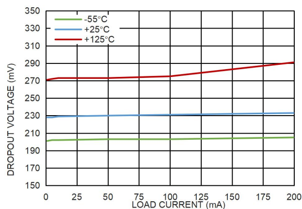
图 12. 压差电压和负载电流的关系, V_{OUT}=5.0V
