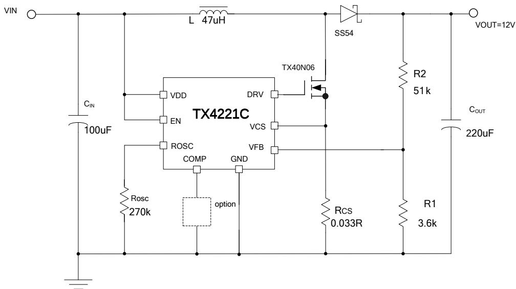
TX4221C典型升压应用电路图
