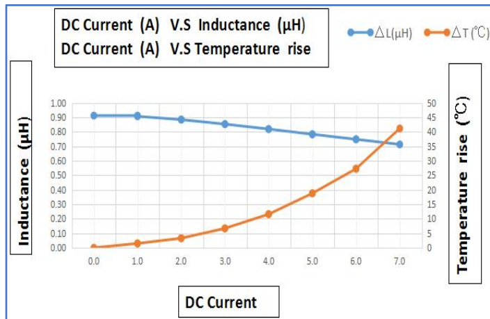
GSM0420-1R0-M
