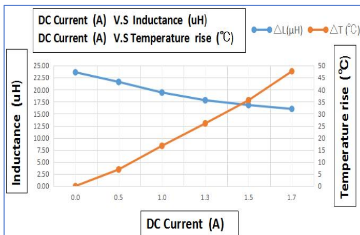
GSM0420-220-M
