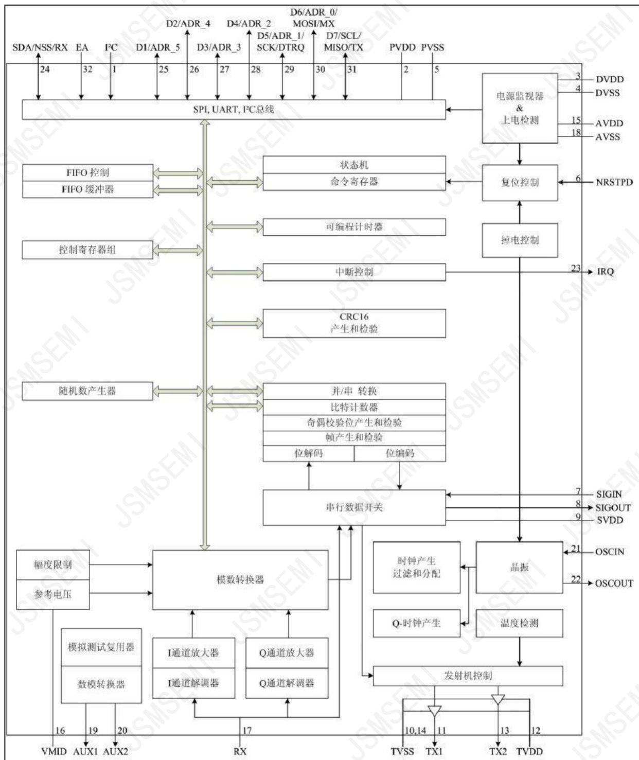
图 2 功能框图
