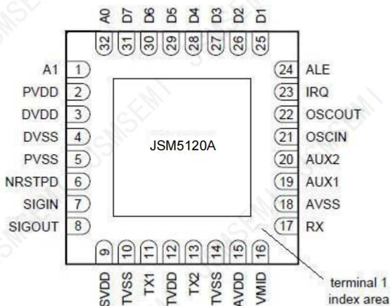
图 1 QFN32 封装管脚图
