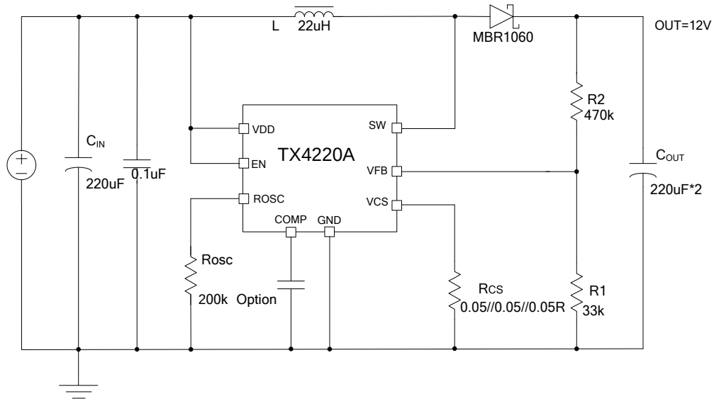
TX4220A典型升压应用电路图
