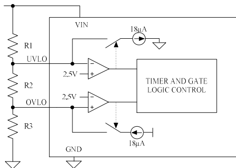
图4 三电阻串联设置过压和欠压保护
