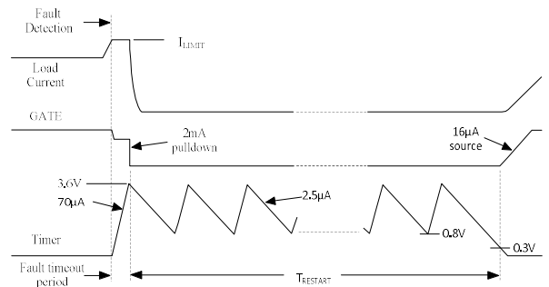
图9 过流保护波形
