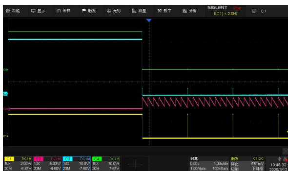
图10 过流保护
