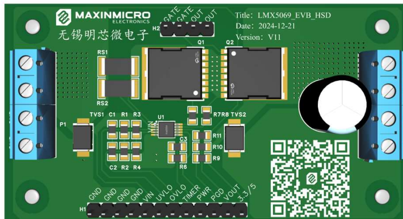
图1 评估板正面
