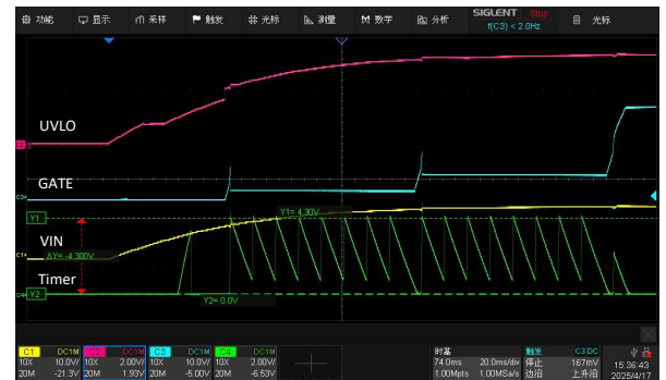
图17 大电解开启时的多次重启波形
