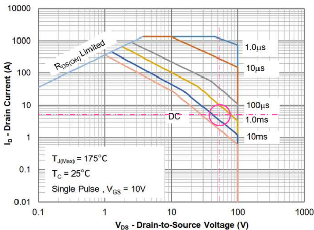
图12 MX10T01AHTL安全工作区示意图
