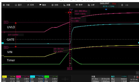
图16 UVLO电阻较小开启过程
