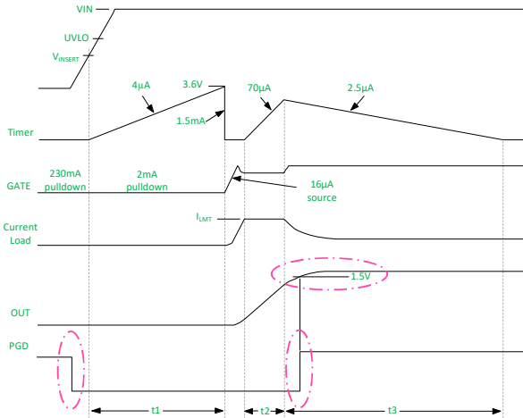
图13 PGD建立示意图
