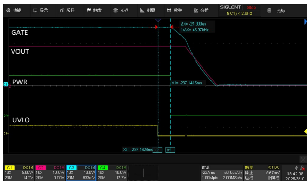
图6 输入欠压保护波形
