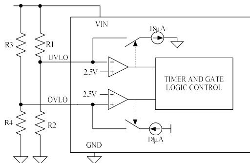
图5 过压和欠压分别设置
