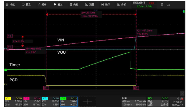
图14 上电过程中的PGD波形
