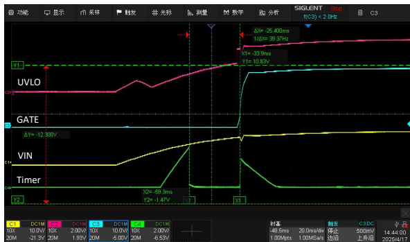
图15 UVLO电阻较大开启过程
