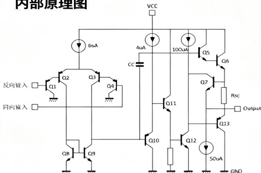
图 1 2904 的内部原理图
