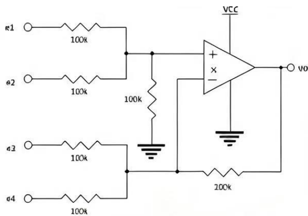
图2 直流加法放大器
