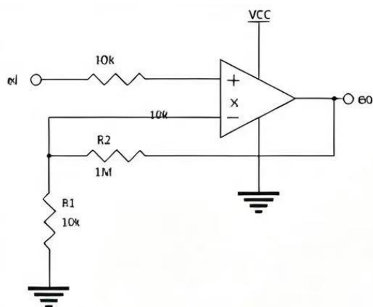
图1 同相直流放大器
