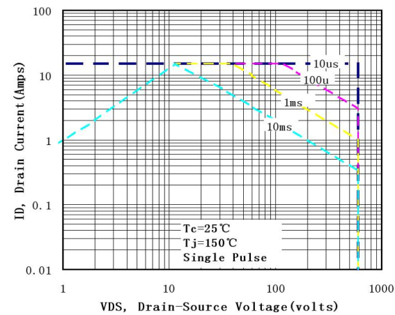
图 8(T0-262&263)最大安全工作区曲线 Fig8 Maximum Safe OperatingArea
