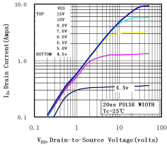
图 1 输出特性曲线, T_c=25^\circ\text{C}
