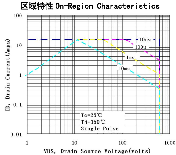
图 6(T0-220)最大安全工作区曲线 Fig6 Maximum Safe OperatingArea
