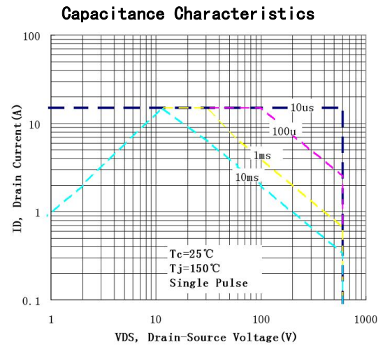
图 7(T0-220FP)最大安全工作区曲线 Fig7 Maximum Safe OperatingArea
