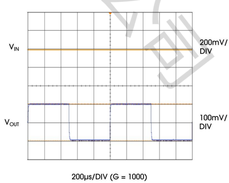
小信号响应 (G = 1000)
