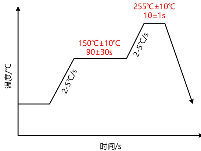
图 23: 焊接温度曲线
