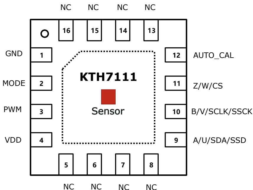
图 3: QFN-16L 3mmx3mm 传感器位于几何中心
