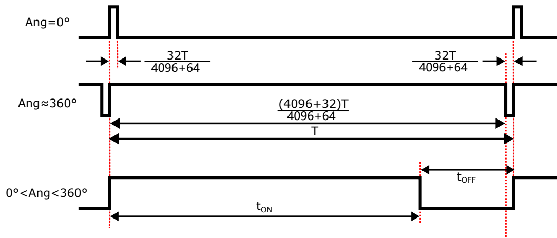
图 18: PWM 时序
