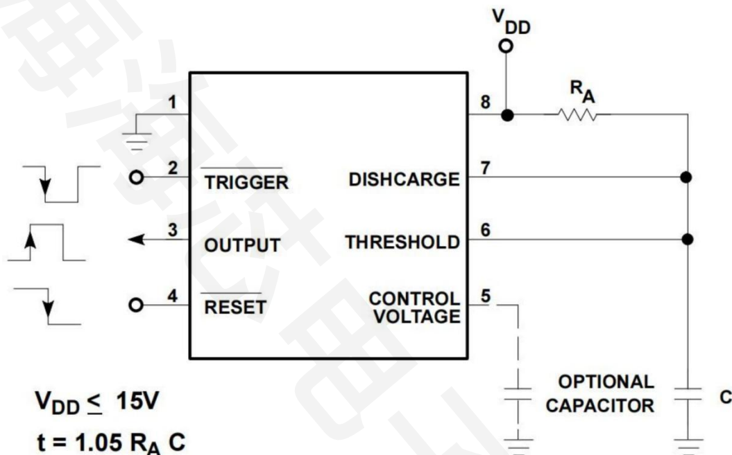
图 1：单稳态（单次）
