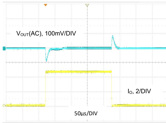
图 15. V_{OUT} = 1.2V , I_O = 0.1A 至 4.5A , FPWM 模式
