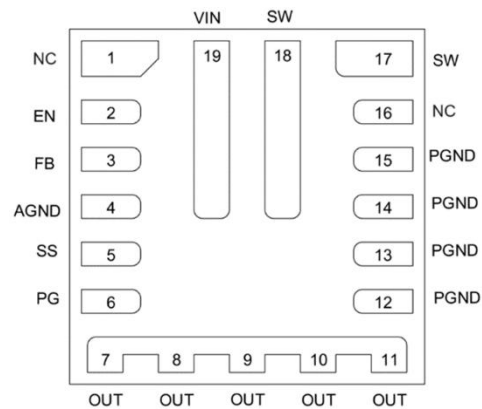
19 引脚 LGA (3mm x 3mm)
