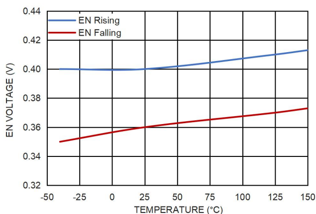
图 10. EN 阈值和温度的关系
